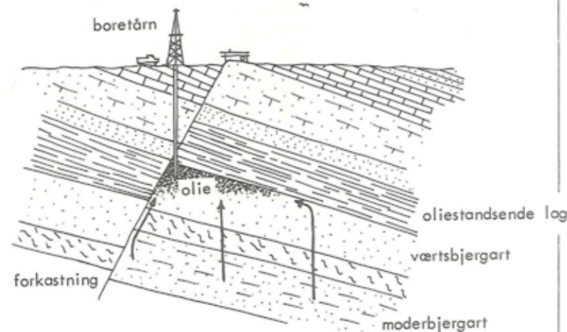
FORKASTNING SOM OLIEFÆLDE
