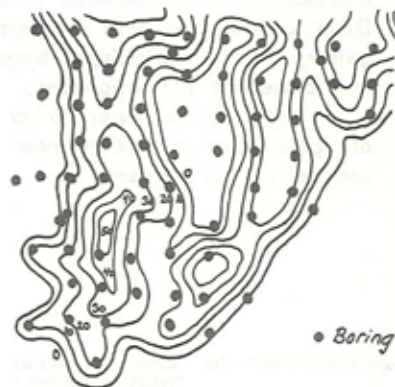
Isopachkort - kort over tykkelsen af f.eks. olieførende sandlag.
