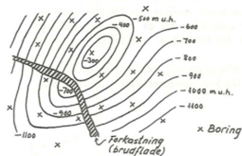
Konturkort - "højdekort" over grænsefladen mellem jura- og kredtlag.
