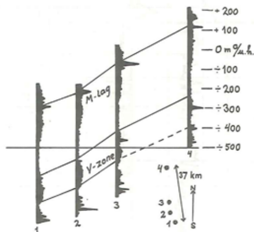
Kurver over elektrisk modstand i 4 borer på strube. Kurven fra en ny (5.) boring mellem 1 og 4 vil sandsynligvis passe ind i skemaet.
