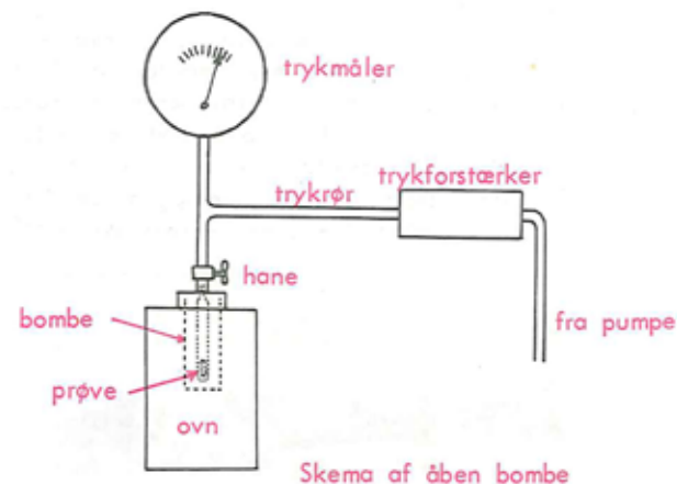
Skema af åben bombe
