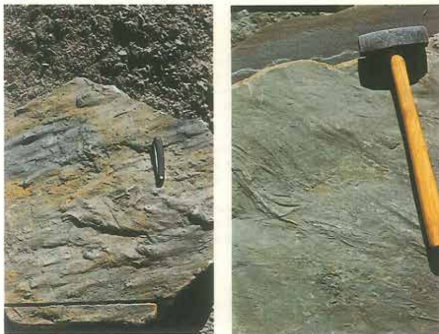
Flysch-lagflader
