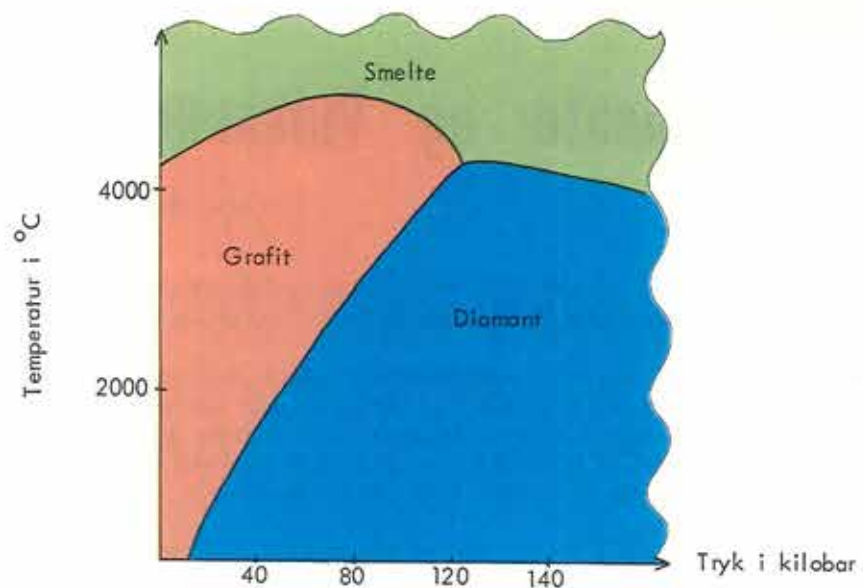
Figur 1. Kulstofs fasediagram. (Efter Fyfe, 1964)
