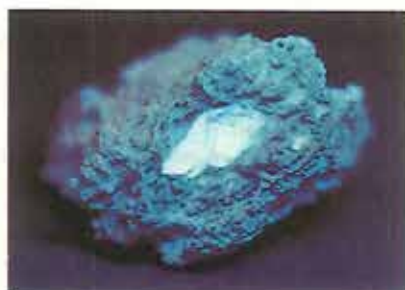
Cølestin-konkretion i UV
