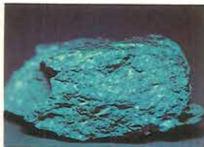
Scheelit i UV
