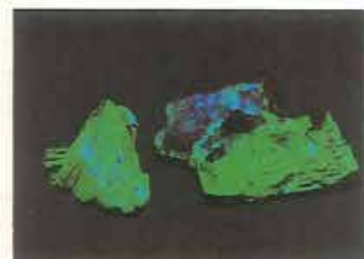
Autunit fotograferet i UV.
