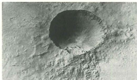
Krater fra underjordisk atomsprængning, cirka 360 m i diameter. Sprængkraften svarede til 100 000 TNT.
