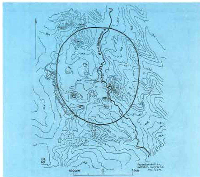
Figur 5. Landskabskort over Nøvling saltdome. Krydset angiver lokaliteten for figur 6. Bemærk det snoede forløb af åen midt i domens samt den stejle skrænt langs saltdomens vest- og sydgrænse.
