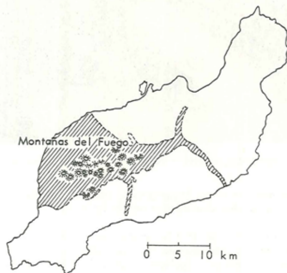
Lanzarote. Det skraverede område dækkes af materiale fra udbrudsperioden 1730 - 36.
