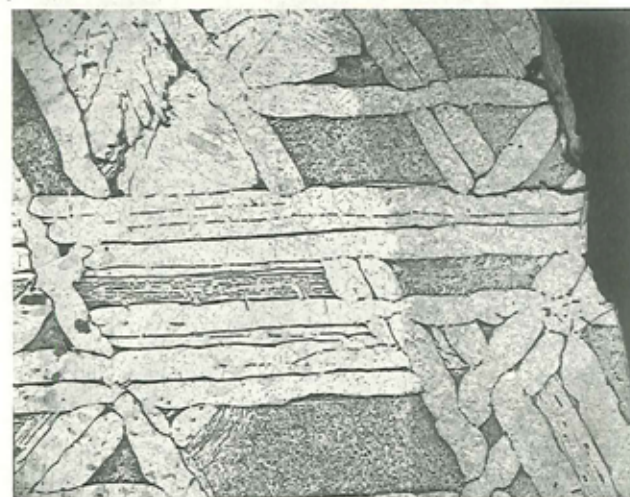
Poleret og ætset snit vinkelret på overfladen af en jernmeteorit med Widmanstättensstruktur. De lyse lameller består af jern med 7% nikkel, mens de mørkere mellemrum har mere nikkel, normalt mellem 10 og 40%. - Yderst til højre er strukturen grå. Denne 2 mm brede zone blev opvarmet til over 750^\circ \text{C} , da meteoriten passerede atmosfæren.
