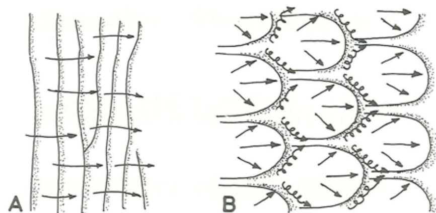
Figur 5. A Parallelle strømrubber, B tungeformede strømrubber. Prikket signatur viser beliggenheden af de stejle læsider.
