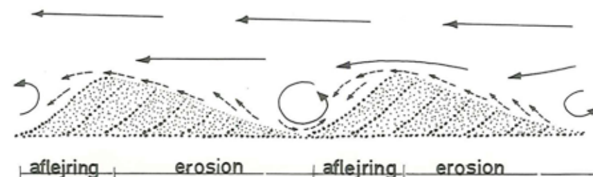
Figur 4. Tværsnit i strømrubber. Fuldt optrukne pile viser vandets strømning (bemærk hvirvlerne i trugene), stiplede pile viser materialetransporten.
