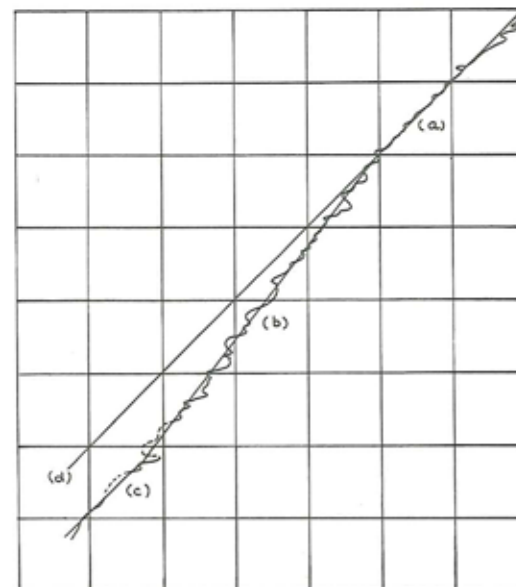
Figur 4. C-14 dateringen af årringe (af "Bristel cone pine" = en fyrre- art) sammenlignet med årringenes korrekte absolutte alder (d). Den bugtede kurve er en tilnærmet kalibreringskurve for C-14 datering. Middelforskellen mellem C-14 alder og træalder er angivet ved de rette linier (a), (b) og (c). (Suess og Tauber).
