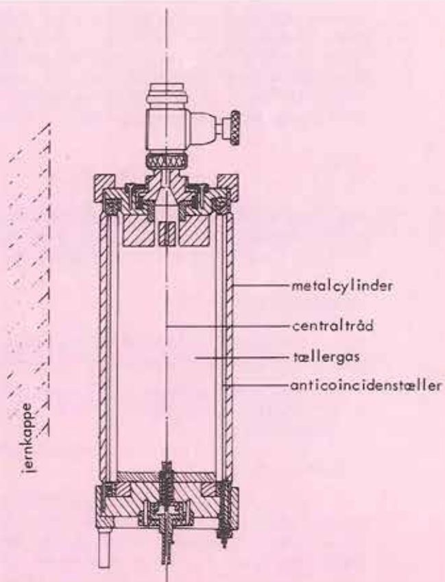
Figur 2. Den principielle opbygning af en C-14 tæller. En 20 cm tyk jernkappe omgiver tælleren for at forhindre de kosmiske stråler i at trænge ind i tælleren og forårsage falske impulser. Da jernkappen imidlertid ikke er i stand til at standse samtlige stråler, er der indbygget en speciel tæller, en antikoincidenstæller, der modvirker registrering af de udefra skabte impulser. (Efter Oeschger).
