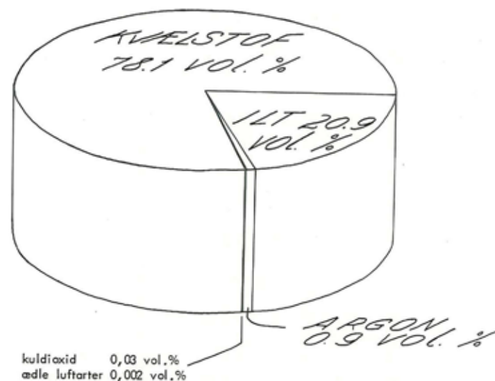
Figur 2. Atmosfærens hovedbestanddele
