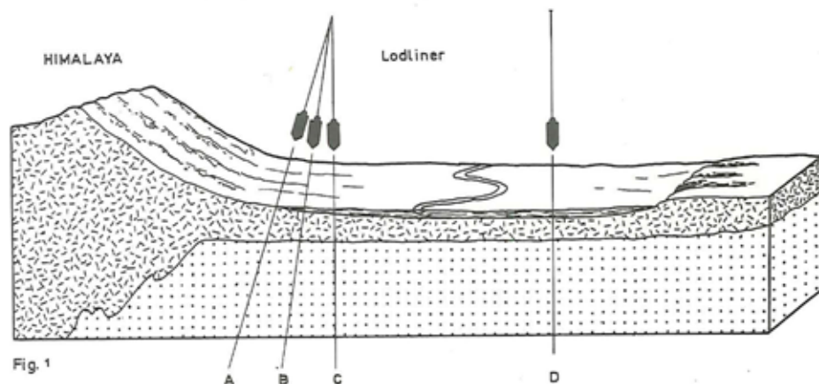
Figur 1. Afvigelser i lodlinens retning ved Himalaya. A: Teoretiske afbøjning på grund af bjergkædens tiltrækning. B: lagttaget afbøjning. C: Ideelle retning uden påvirkning af omgivende masser. Den ringe afbøjning må skyldes, at bjergenes overjordiske masseoverskud opvejes af dybtgående "rødder" af lette bjergarter.
