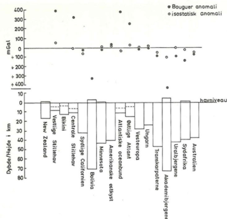
Figur 6. Tykkelser af jordskorpen sammenholdt med Bouguer anomalier og isostatisk afvigelser målt i mGal.
