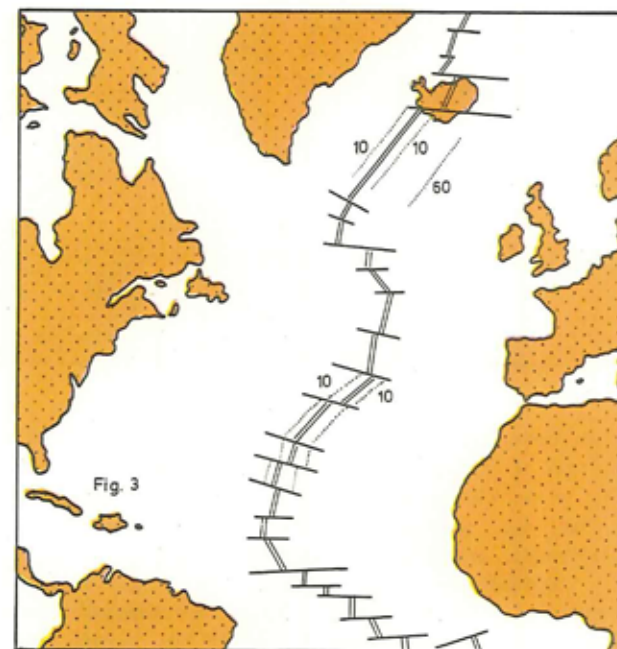
Figur 3 viser, hvordan en del af den midatlantiske ryg forløber i detaljer. Man ser, at Island ligger midt over ryggen, og man skulle derfor vente, at man på Island direkte kunne måle pladernes bevægelser. Det har
