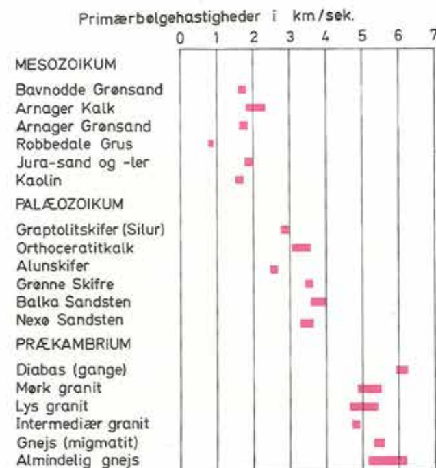
Figur 9. Seismiske chokbølgehastigheder i bjergarter fra Bornholm.
