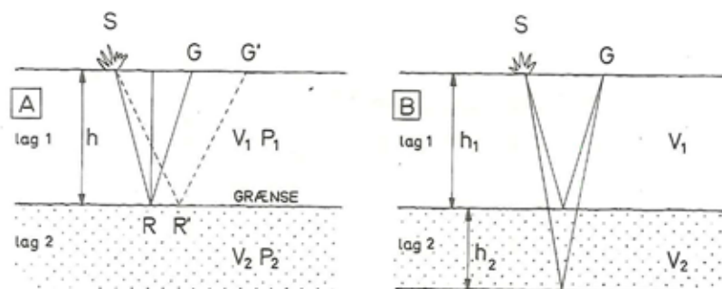
Figur 6. Principper i målinger ved den seismiske refleksionsmetode (tilbagekastning). A: Forholdene ved en enkelt reflekterende grænseflade. B: To reflekterende grænseflader. V_{1-2} = Den seismiske hastighed i de pågældende lag. P_{1-2} = Vægtykkelser af de pågældende lag. h_{1-2} = lagtykkelser. S = sprængsted. G = Geofon.
