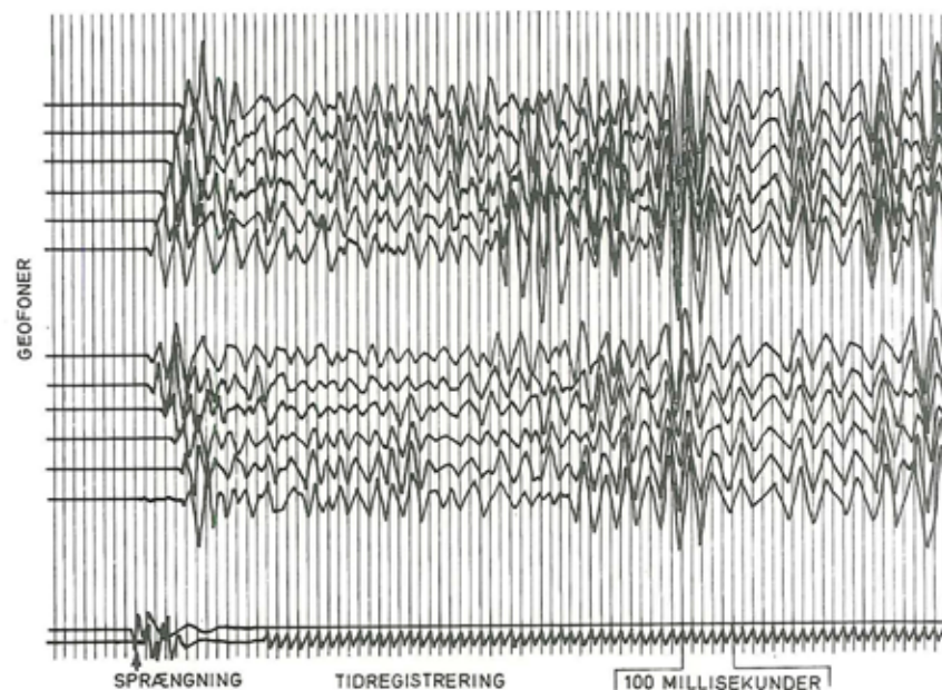
Figur 7. Typisk reflektionsseismogram optaget af en recorder med indgange for 12 geofoner.
