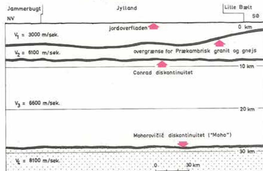
Figur 5. Strukturforholdene i den dybere jordskorpe i et nordvest-sydøst profil gennem Jylland fra Jammerbugt til Lille Bælt. For at fremhæve de små højdeforskelle er dybdelestokken forstørret 5 gange. Diskontinuiteter er grænser, hvor der sker springvise ændringer af de seismiske hastigheder, fordi bjergarterne får en anden sammensætning. Mohorovičić diskontinuiteten, der for nemheds skyld internationalt ofte bare betegnes som "Moho", repræsenterer grænsen mellem Jordens skorpe og kappe.
