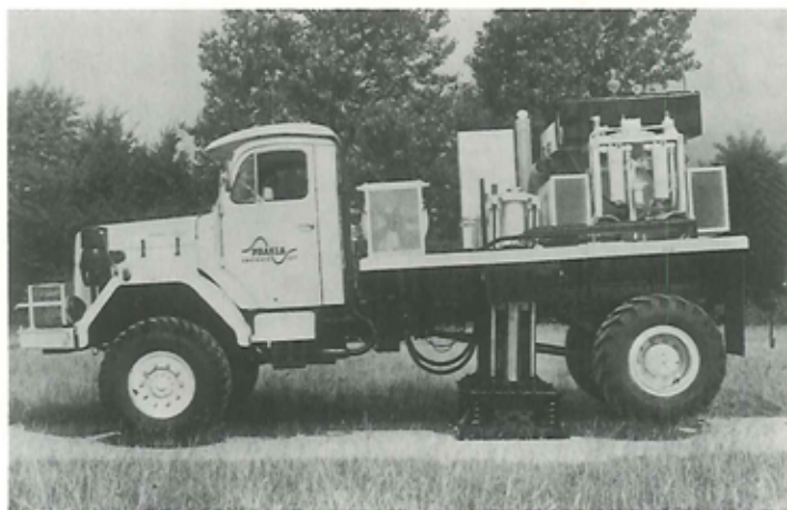
Figur 10. Med en passende stor energi kan en vibrator monteret på en lastbil frembringe en kontinuert serie chokbølger til seismiske undersøgelser af den højereliggende undergrund (Firmaet Prakla, Vesttyskland).
