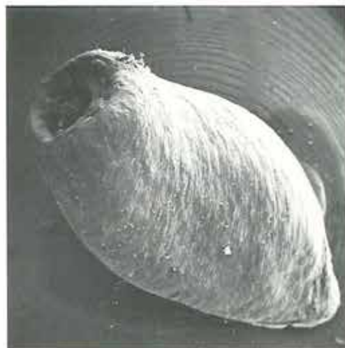
Figur 4. Frø af Spirematospermum wetzleri, forstørret cirka 10 gange
