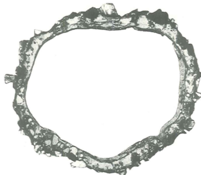
Figur 3. Lyrør fra Herning set i tværsnit. Min.Mus.Saml. Den indre diameter måler 6,5 \times 5,5 mm. Rørets glasmasse er tydeligt tyndere end i lyrrøret fra Lüneburg - 0,5 mm - og det indeholder flere ikke-smeltede mineraler. Mikrofoto uden polarisator (M.Ghisler).
