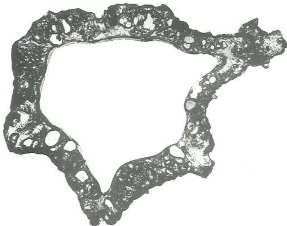
Figur 1. Lynør fra Lüneburger Heide set i tværsnit. Min.Mus.Saml. Den gennemsnitlige indre diameter er cirka 6,5 mm. I rørvæggens glasmasse ses luftbobler og enkelte ikke-smeltede mineralgrain. Mikrofoto uden polarisator (M.Ghisler).
