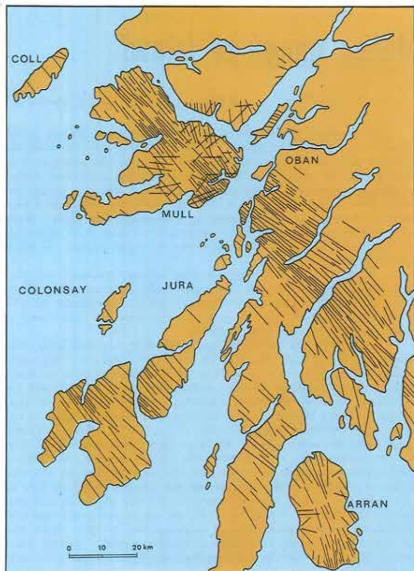
Figur 1. Vulkan-plutonkompleks på øerne Mull og Arran i Vestskotland, præget af gangsværme.
