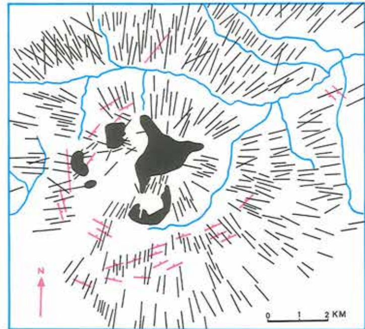
Figur 3. Radiale gange og keglegange ved "The Sunlight District" i Wyoming, USA.
