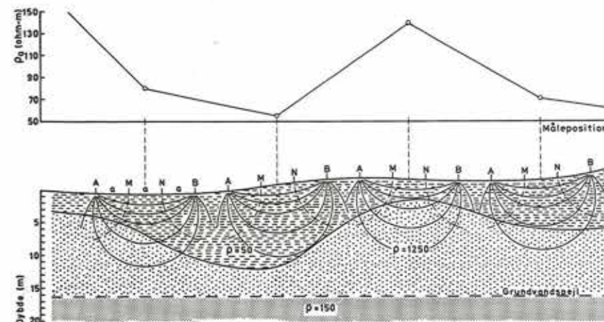
Figur 4. Linieprofilmåling: Den tilsyneladende specifikke modstand \rho_s varierer med tykkelsen af moræneleret, der dækker de tørre grusaflejringer.
