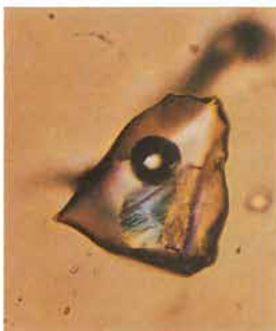
Indeslutning med væske, gasboble og to dattermineraller. Kvarts fra Evje pegmatit, Sydnorge. Forstørret 25 gange.
