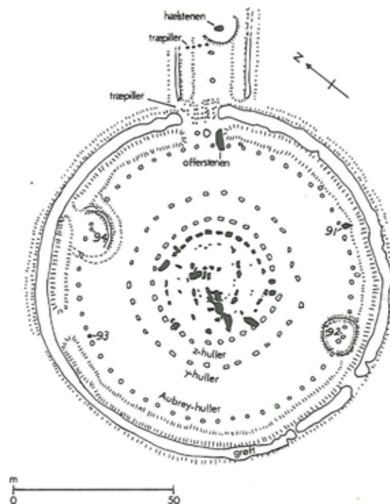
Plan over Stonehenge, med ikke synlige træpiller, stenhuller og Y og Z huller indtegnnet. Eksisterende sten er farvet sorte.
