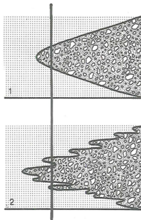
Figur 3. Øverst: Principskitse visende lagfølgen smeltevandssand, moræner og smeltevandssand (en "kineto-stratigrafisk enhed") fra ét isfremstød.
