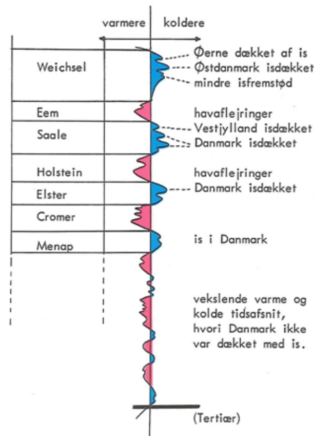
Figur 2. Stærkt forsimplet kurve over klimasvingningerne i Kvartær-tiden. Kurven er ikke målestok-tro.
