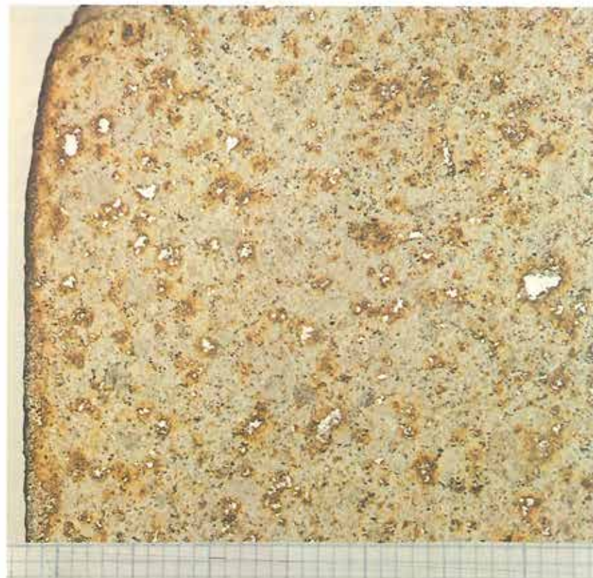
Figur 4. Nærbillede af en snitflade gennem Ella Island chondriten vinkelret på overfladen. Den mørkebrune smelteskorpe er cirka 1 mm tyk. Spredt i den finkornede, grå grundmasse ses dels de skinnende metalkorn omgivet af en rustfarvning, dels de mørkegrå og lysegrå runde chondrer af nogle få millimetres størrelse. (Målestokken er inddelt i millimetre).
