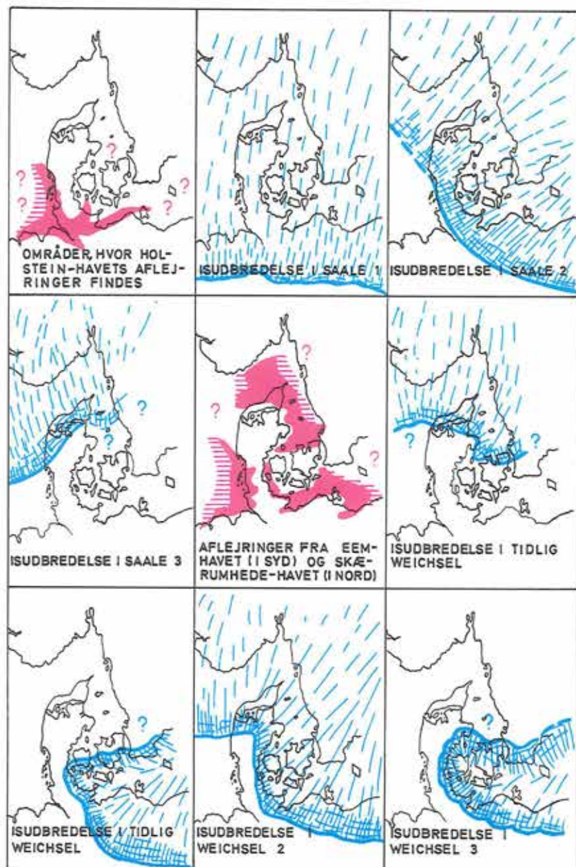
Figur 1. Forskellige isstrømmes omtrentlige udbredelse i de sidste to "is-tider", samt kort over kendte havudbreddelser i de to sidste mellemistider.
