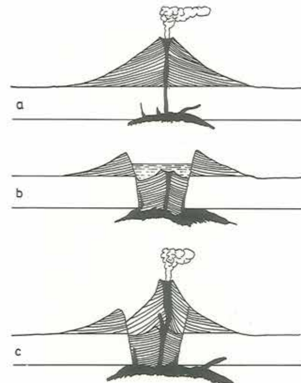
Figur 6. a: en keglevulkan (stratovulkan) er bygget op. b: i denne vulkan har en caldera indsykning fundet sted og en sø er dannet i calderaen. c: en ny stratovulkan er under opbygning (situationen svarer til Somma-Vesuv's udseende i dag).
