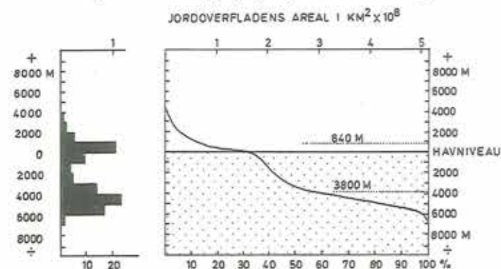
Figur 1. Den procentvise arealfordeling af jordoverfladen - til venstre vist som søjlediagram og til højre som en kumulativ, hypsometrisk kurve. Landområdernes middelhøjde er 840 m, og middelhavdybden er 3.800 m.
