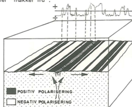
Figur 5. Skematisk snit gennem oceanbund dannet ved seafloor spreading udenom en midtoceanisk ryg. Den magnetiske feltkurve (øverst) varierer symmetrisk og i takt med den skiftende polarisering af oceanbunden.
