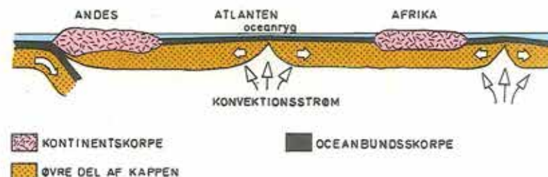
Figur 4 viser et lithosfæretværsnit. En opadgående konvektionsstrøm under den midatlantiske ryg bringer smeltet magma op til overfladen hvor ny oceanbund dannes for derefter at transporteres væk. I dybgraven udfor Andeskæden "konsumeres" havbund i samme tempo som denne nydannes andetsteds.
