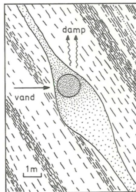
Figur 6. Skematisk lodret snit gennem en Oklo-reaktor. Med stregsignatur er vist diverse sandsten, mens prikssignatur viser uranmineraliseringen (tættere prikning = højere koncentration). Reaktionen kunne kun ske, hvor uran-koncentrationen var over 10%. Reaktorzone er vist med en cirkel. Da uranåren er mere end 0,5 m tyk, er de langsomme neutroner blevet indfanget af indholdet af Uran-235 inden de nåede ud i sidestenen. Grundvandet fungerede som moderator, og når temperaturen i reaktoren nåede vandets kogepunkt, fordampede noget af vandet til der var balance mellem varmeafgivelse til omgivelserne og varmen fremkommet ved reaktorprocessen.
