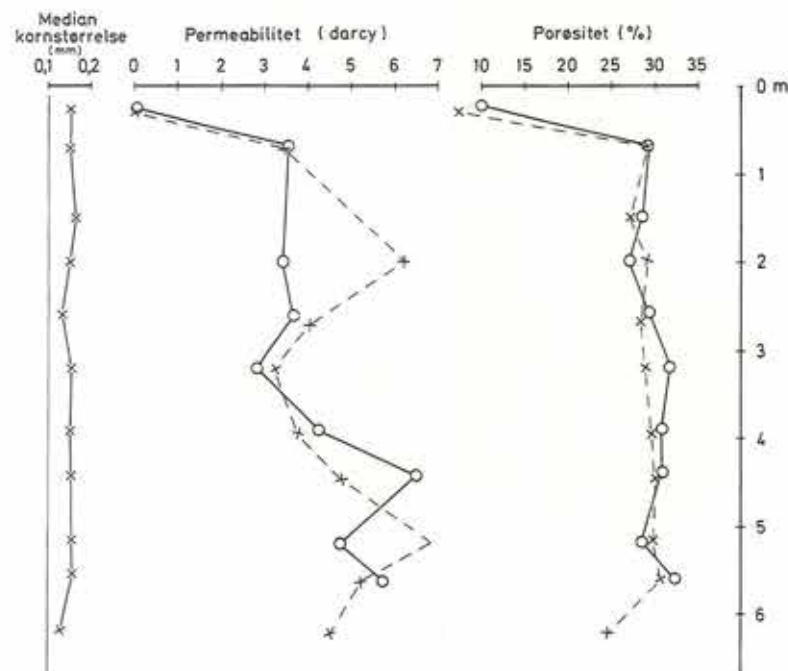
Figur 6. Porøsitet- og permeabilitetsværdier fra laboratorieundersøgelse af sandstenskerne fra Gassum Formationen. Darcy er en måleenhed for permeabilitet baseret på hastigheden af passage af 1 cm 3 vand ved 1 atmosfæres tryk gennem et porøst medium med tværsnitsarealet 1 cm 2 og højde 1 cm. Toppen er kalkspatcementeret, hvilket tydeligt afspejles i de målte værdier. Vertikal porøsitet og permeabilitet er markeret med cirkler, horisontal med stjerner (efter Holm & Priisholm 1978).
