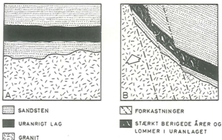
Figur 5. Koncentration af Uran-235 ved Oklo. A: Efter udfældning af uranmalmårene i sandlagene dækkedes det hele af sand. B: Graniten vest for legemet blev skudt op, hvorved malmforekomsten fik en betydelig hældning og samtidig blev gennemsat af revner og sprækker. Grundvand sivede gennem sprækkerne og opløste uranet, som blev genafsat som stærkt beriget malm i årer og lommer andre steder i malmlegemet.
