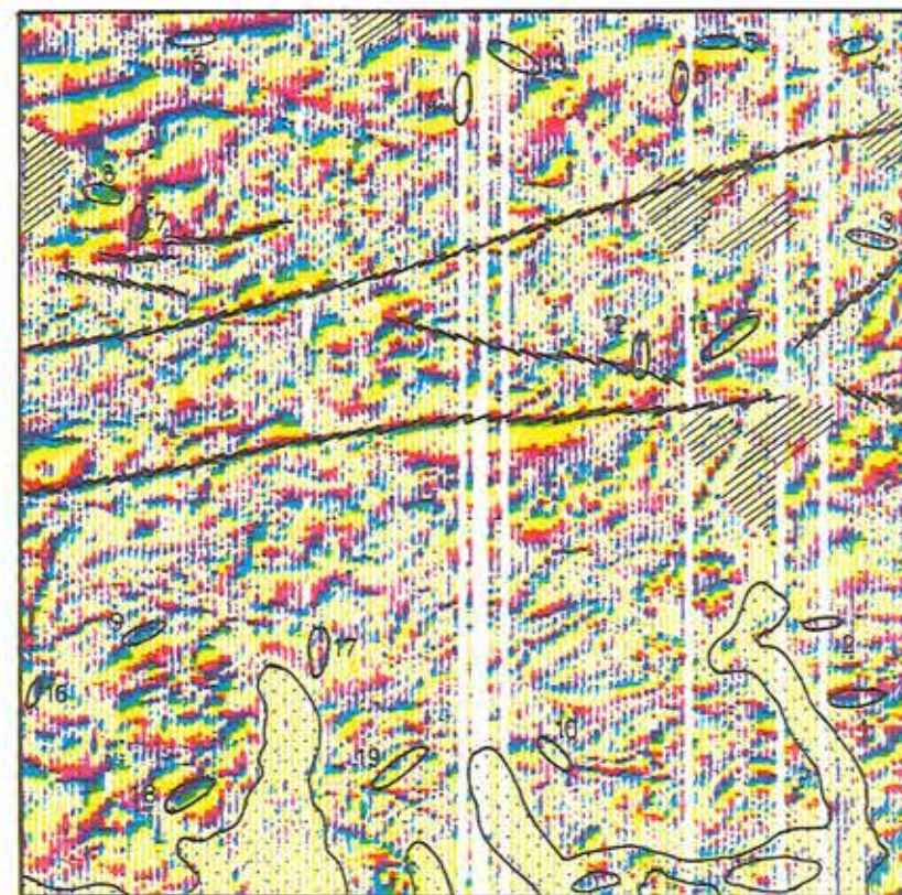
RAMA-kort visende de radiomagnetiske anomalier i et 25 x 25 km stort område ved Enköping. Anomalierne markeres af skift fra stærke til svage farver og tætliggende farver. Mange anomalier forårsages af grundvandsførende sprækkezoner. Zigzaglinier viser el-ledninger m.m., prikkede områder er søer, og større lerdækkede områder er skravet. Numrene viser de undersøgte anomalier.
