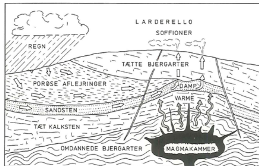
Figur 2. Schematisk snit visende den geologiske baggrund for det geotermiske system i Larderello-området. Se iverigt teksten.
