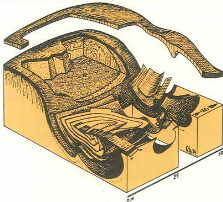
Figur 6. Blokdigram der viser den strukturelle opbygning af Præstebjerg. Sammenlign med figur 5.
