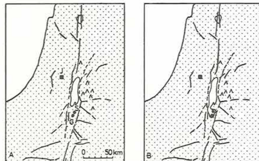
Figur 2. Fortid og nutid i Jordandalen. A: ca. 2000 år f.Kr. B: Nutid. Byerne Sodom og Gomorra blev antagelig oversvømmet af Dødehavet i forbindelse med forkastning og kipning mod syd af Jordandal-blokken mellem forkastningerne. S = Sodom. G = Gomorra. J = Jerusalem. Streger viser forkastninger og vinkler angiver vulkaner.
