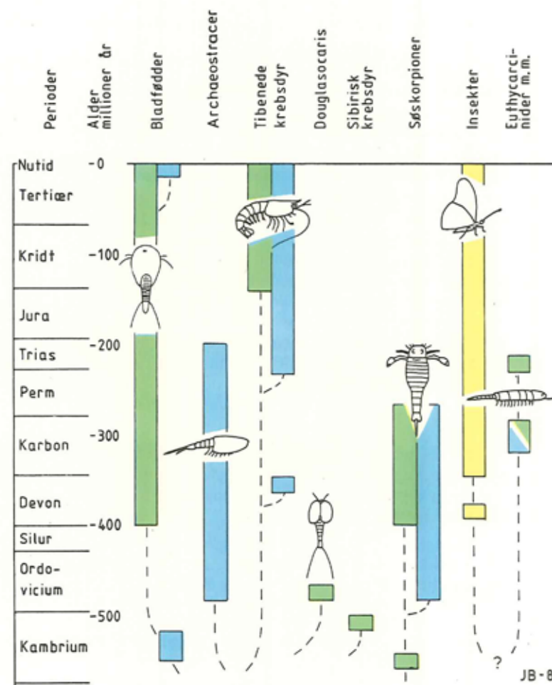
Figur 1. Den kendte geologiske udbredelse af nogle udvalgte leddyrgupper. Blå farve viser forekomst i havet, grøn farve forekomst i ferskvand og gul farve liv på land. En levevis i ferskvand eller på land, hvor mulighederne for fossilbevarelse er temmelig ringe, kan let give store huller i den tidsmæssige udbredelse.
