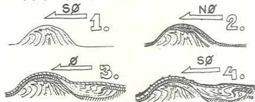
Figur 5. Fire trin i Præstebjergs udviklingshistorie. Pilene angiver hvorfra de forskellige isfremstød kom. Skråkravering er signatur for moræneler.
