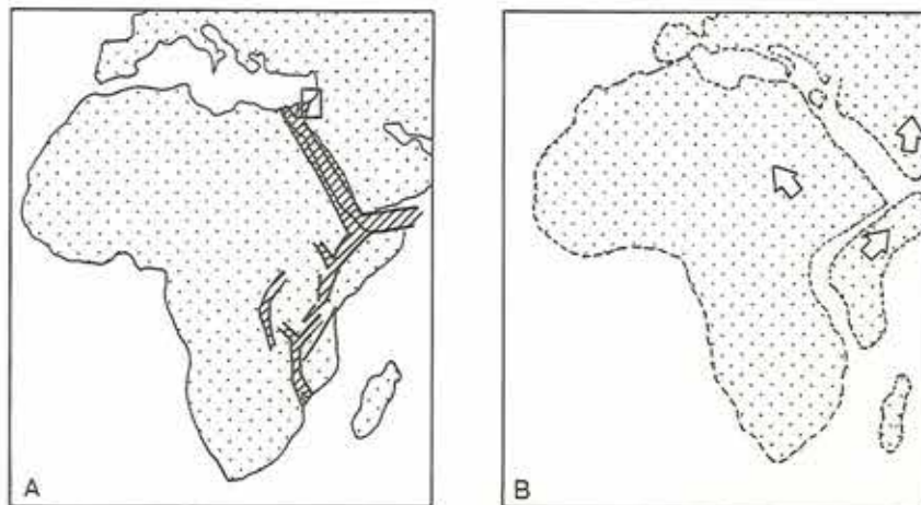
Figur 3. Det østafrikanske Rift-system (skraveret i figur A) - stedet for en igangværende opsplitning af kontinentet. Det indrammede område er vist i figur 2. B: Om 50 millioner år ?
