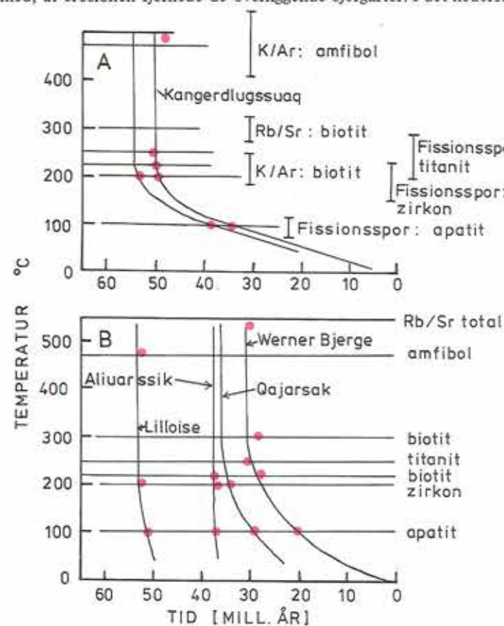
Figur 3. Diagrammer visende afkølingsforløbet for de daterede tertiære intrusioner. Øverst (A) intrusioner fra domens centrale del, nederst (B) fra domens ydre del. Efter Brooks og Gleadow (1979). Tid i millioner år.
