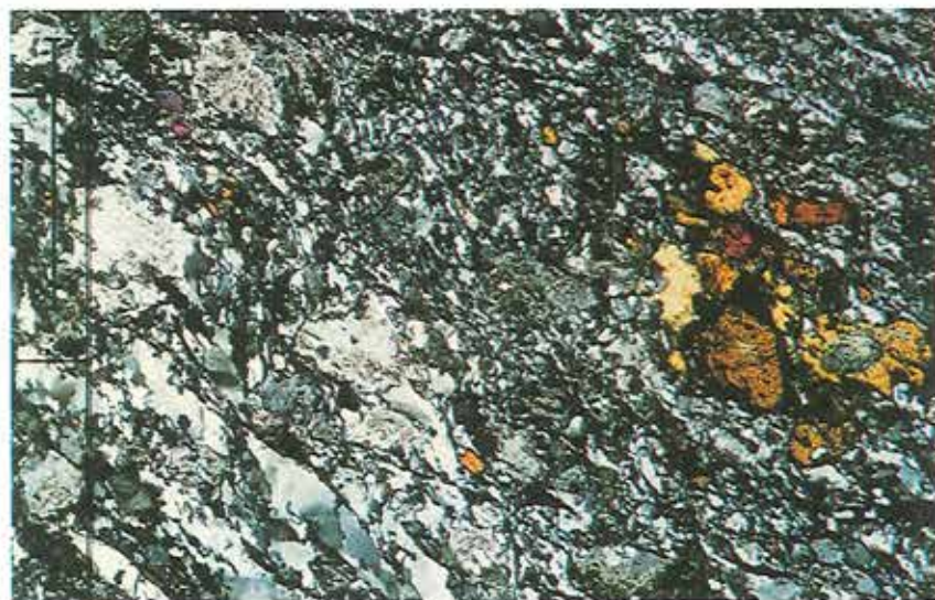
Figur 5. Tyndslib af mylonit dannet ud fra en tonalitisk gnejs. Foruden det fin-kørnede materiale ses lange udvalgte kvartskorn, som internt er opdelt i subkorn. De farvede korn er epidot, som er mere modstandsdygtige overfor mylonitiseringsprocessen. Lok nord for E 18 nær rigsgrænsen mellem Norge og Sverige.
