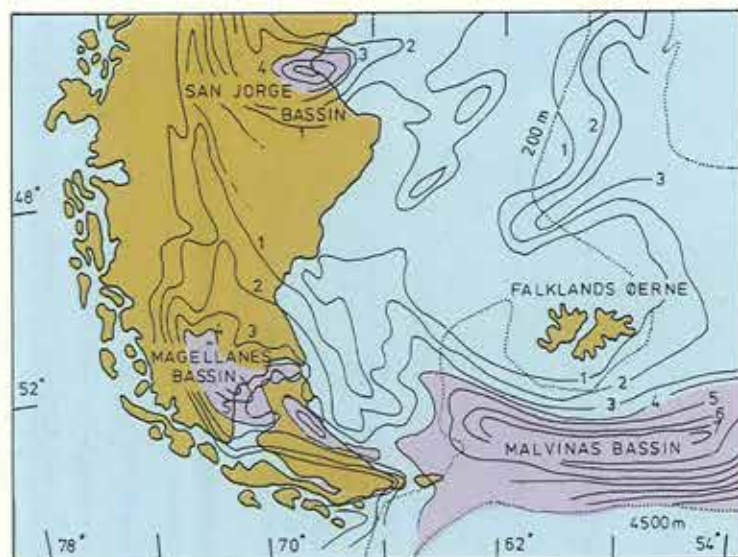
Figur 4. Ekstracordilleriske bassiner i Sydatlanten. Fuldt optrukne linier viser dybde i km til det prækambriske underlag. Punkterede linier viser havdybde i meter.
