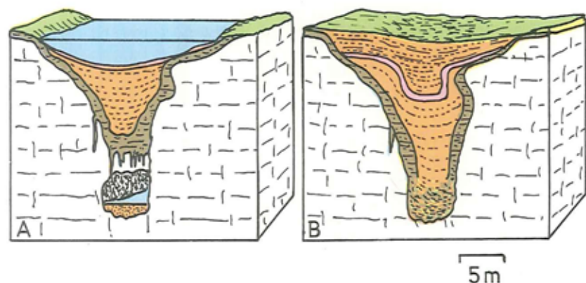
Figur 5. Model for dannelsen af en karstbetinget dal ved Ålborg. Til venstre ses et søbassin eller flodløb, hvor et silt-lag er aflejret ovenpå lagdelte sand. I Kridtet under disse aflejringer findes en karsthule med eget vandspejl og sedimentation.
