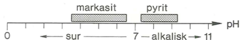
Figur 5. Markasits og pyrits afhængighed af surhedsgraden (pH) i omgivelserne ved udfældning fra opløsninger. Er omgivelserne sure (syre-agtige) udfældes fortrinsvis markasit, mens pyrit hovedsagelig fældes fra alkaliske opløsninger.
