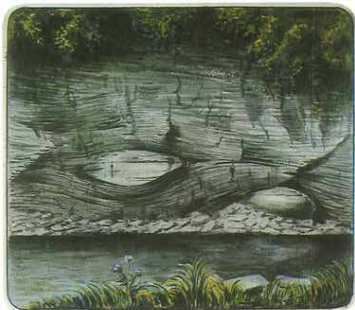
Altinskifer med Antrakonit-Boller ved Læså
