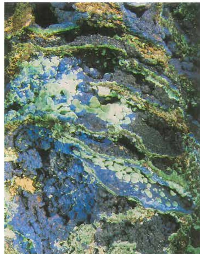
Kobberminerale Azurit (blå) og Malachit (grøn) fra Bisbee, Arizona, U.S.A. ca. 3 x naturlig størrelse. Billedet er (som forsidebilledet) hentet fra Ole Johnsen's bog: Mineraler, form og farve.
