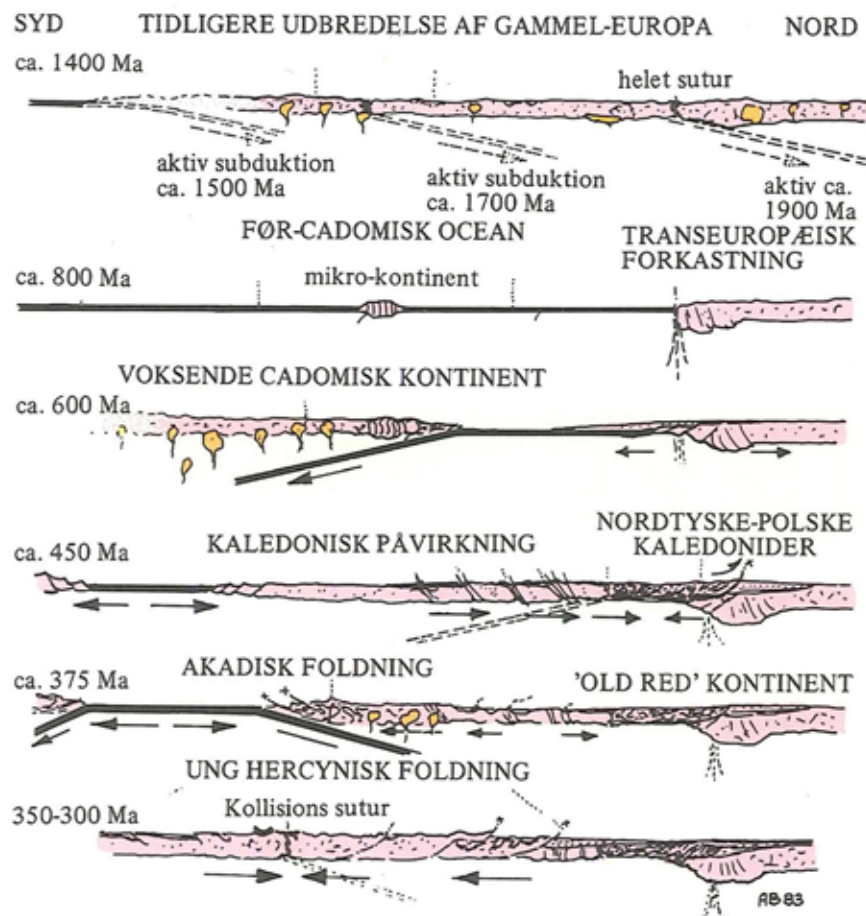
Figur 5. Pladetektonisk model for kontinentalskorpe udvikling i Europa (1900-300 millioner år). Efter dannelsen af den Transeuropæiske Forkastning (ca. 800 mill. år), opbygges en ny kontinentalskorpe i Mellemeuropa i forbindelse med den Cadomiske, Kaledoniske og Gammel (=Akadisk) og Ung Hercyniske foldning.
