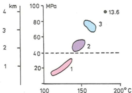
Figur 8. Kvartskrystallernes dannelsesbetingelser.
