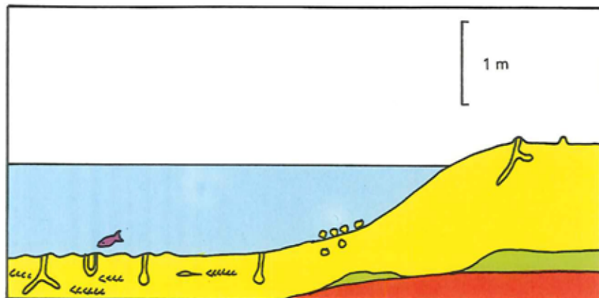
Figur 4. Skematisk tværsnit gennem sandfladerne i midten af Ras al Hamra bugten. Med gult er vist kalksand med spredte grave gange efter krabber. Grønt viser æolisk sandsten af Kvartær alder, og orange angiver den tertiære Umm er Radhuma kalksten.
