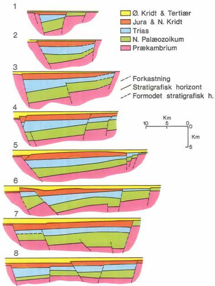
Figur 1. Øst-Vest - gående profiler gennem Rønnegraven. Profilerne placering fremgår af figur 2.
