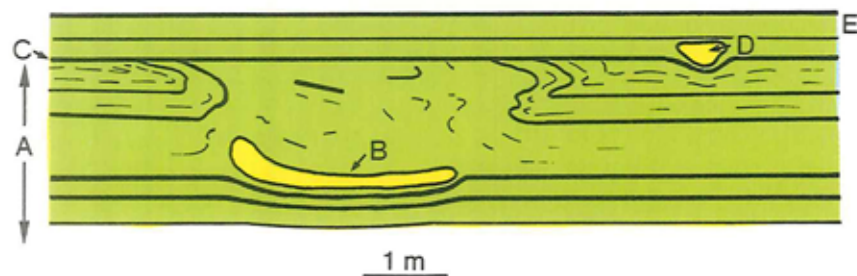
Figur 6. Skitse af lokalitet visende "slump"-struktur. Itubruddt, foldet og sammenfalden lagdeling (A) omkring xenolit B. En anden mindre xenolith D har trykket det underliggende lag C lidt ned, medens de senere lag E er uforstyrrede. Lagene hælder ca. 30^\circ , så deres reelle tykkelse er ca. 20 % mindre end vist på skitsen.
