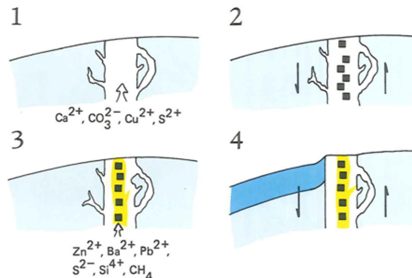
Figur 6. Forenklet fremstilling af dannelseshistorien (fra 1 til 4) for den undersøgte kalkspatåre. 1: Varmer opløsninger indeholdende de viste stoffer (blandt andet kobber) afsætter kalkspat (vist med hvid) i en grå dolomit (lys blå). 2: En forkastning sker langs kalkspatåren og skaber en brecciering, knusning, (vist med sorte firkanter), af den centrale del af åren. 3: Senere opløsninger indeholdende andre stoffer afsætter zinkblende (vist med gul) i den centrale del af åren og langs små sprækker. 4: Kalkspatåren som den ser ud i dag. Vist med mørk blå ses en nedforkastet, oprindeligt højere liggende mørk dolomit.
