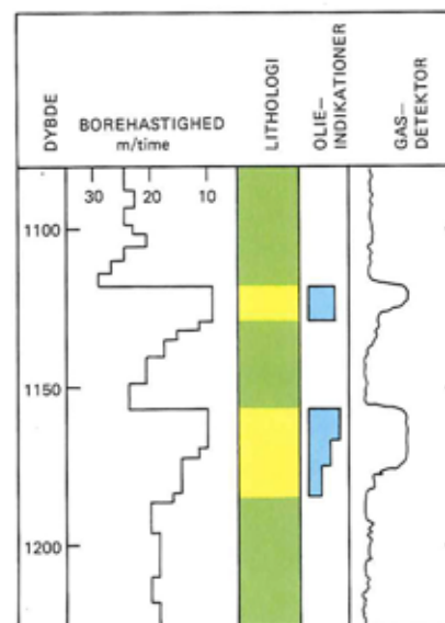
Figur 3. Eksempel på 'mudlog'. Resultaterne af undersøgelserne af boremuddret fra de forskellige boreddybder er vist sammen med lithologien af de lag, der gennembores. Med grønt er angivet skifre, med gult sandsten.
