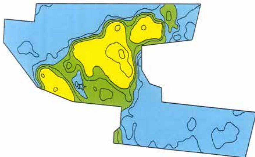
Figur 3. Iso ohm-m kort over det undersøgte område ved Himmelev. Værdier under 80 ohm-m er vist med blå, værdier mellem 80-120 ohm-m med grøn og værdier over 120 ohm-m med gult. Masterhøj er vist med en stjerne.
