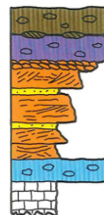
Figur 6. Skematisk lagsøjle fra Himmelev området.
