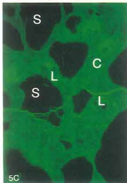
Figur 5. Tyndslidsbilleder af revnet beton. A: set i almindeligt gennemfaldende lys. En revne ses på grund af limens indhold af gult farvestof. Tæt ved revnen ses en farveændring i pastaen, der her indeholder mere farvestof. I to luftporer ses radiært stillede nåleformede krystaller. B: samme udsnit set i polariseret lys med gipsblad i strålegangen. Der ses en forskel i formen på CH-kornene i den smalle omdannede zone om revnen sammenlignet med den uomdannede pasta. De radiært stillede krystaller kan identificeres som Aft-fase. C: Samme udsnit set i fluorescerende lys. Ændringen i porositeten af den omdannede pasta træder nu tydeligere frem. S=sand, C=cementpasta og L=luftporer. Format: 1.08x0.75 mm.
