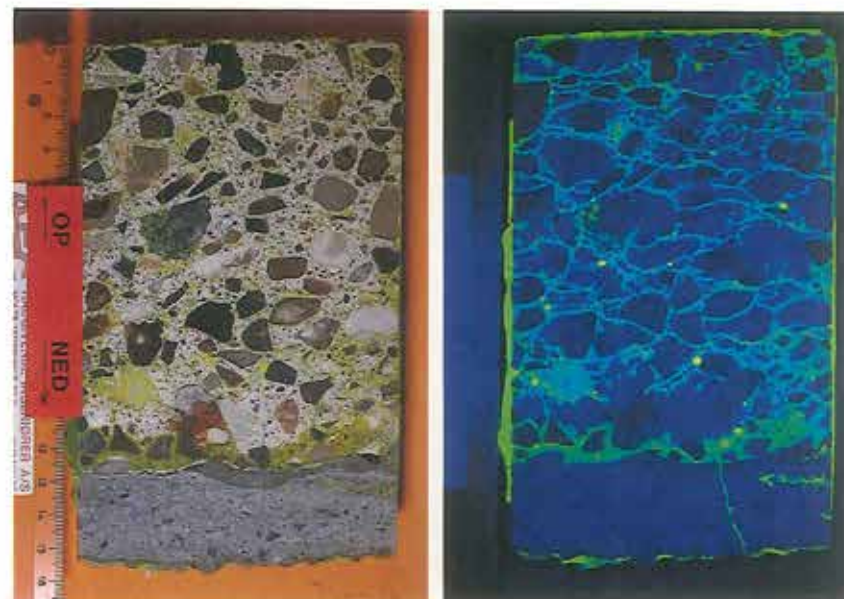
Figur 4. Planslib af borekerne af beton fremstilles ved at save kærnen igennem i midterplanet og polere skæresliden. Herefter imprægneres fladen med et farvestof. Til venstre ses kærnen i almindeligt lys, til højre i ultraviolet lys, hvor farvestoffet får revnebilledet til at træde tydeligt frem.
