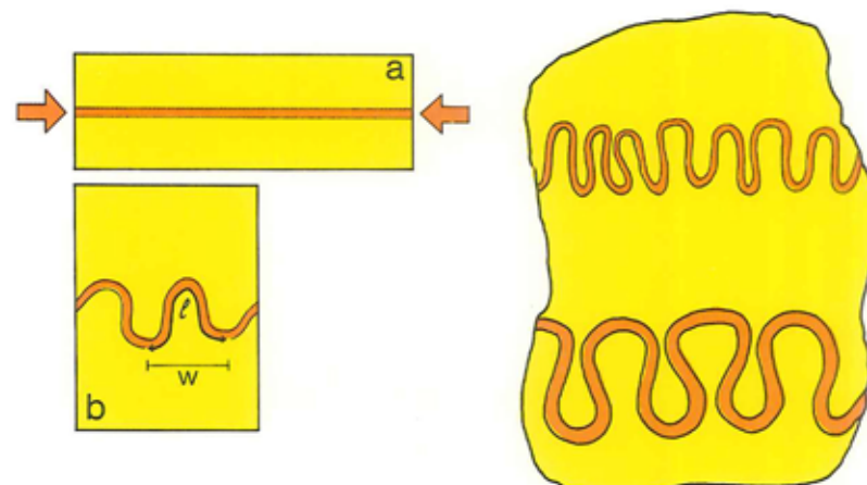
Figur 4. Dannelsen af en ptygmatiske fold ved kompression. I (b) er foldens længde l og bølglængde w angivet.
