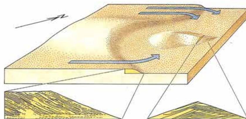
Figur 7. Skematisk tegning fra fronten (læside) af barre B med det højere midterparti og de to afbøjede strømretninger, der opbygger en lang, lav sandtunge foran barren B. Detailtegningerne viser dels snit gennem sandtungen vinkelret på strømmens retning, og dels et snit gennem barren parallelt med strømretningen.
