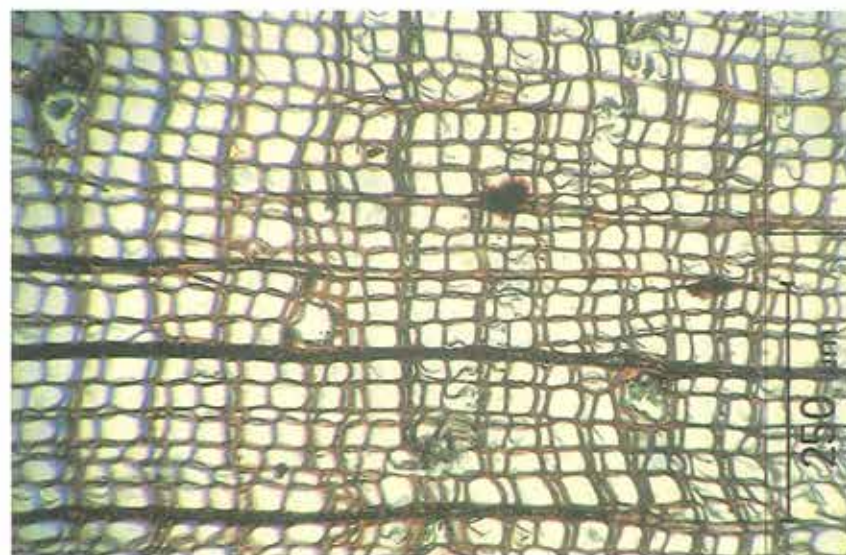
Figur 3. Mikroskopbillede af tværsnit af lærkeved med meget små ringe, der hver for sig kun består af 2-3 lag celler. Der ses også enkelte harpikskanaler.
