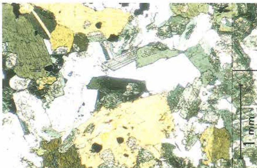
Figur 7. Tyndslidsbillede af diorit. De store grønne og gullige korn er hornblende (amfibol), medens de hvide korn er feldspater og kvarts.
