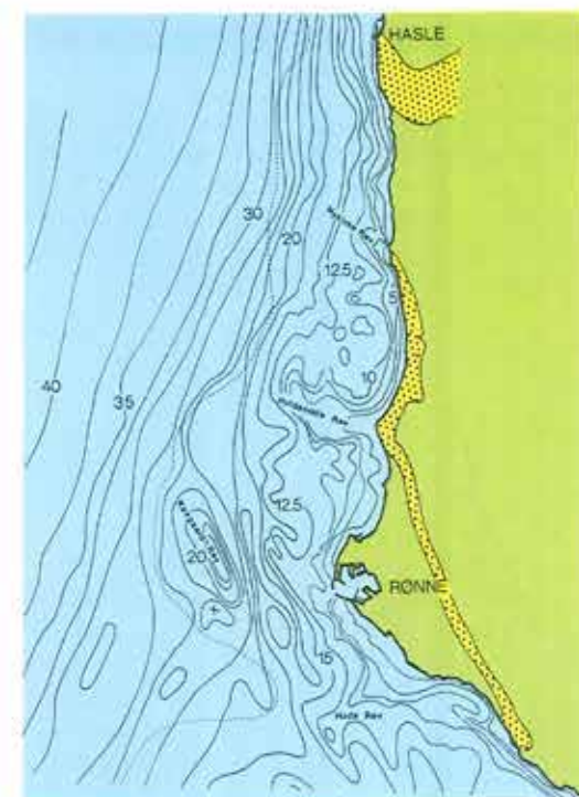
Figur 3. Dybdeforhold vest for Bornholm. Ekvidistansen er 2.5 m og tallene angiver dybder i meter. På kortet ses en tydelig sammenhæng mellem odderne langs kysten og Hasle Sandstenen (gult med prikker). Sandstenen fortsætter ud i vandet som revdannelser (Nykirke Rev og Hvidodde Rev).
