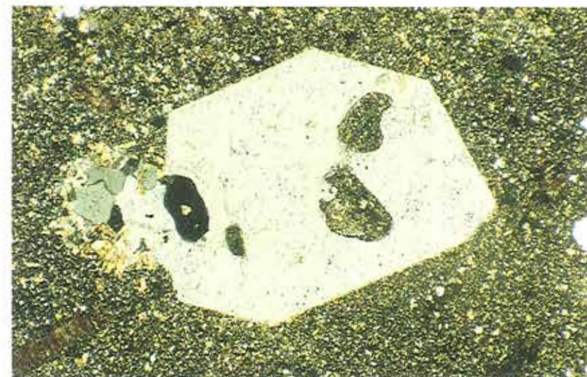
Figur 4 Tyndslibsbillede af en rød østersø-kvartsporfyr (en rhyolit). Der ses en meget stor krystal af kvarts.
