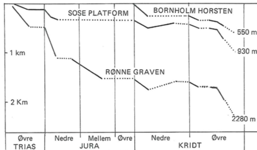
Figur 24. Indsynkningskurver for Bornholm Horsten, Sose Platform og Rønne Gravens østlige del. Kurverne er tegnet på grundlag af aflejringerne nuværende tykkelse, så kurverne 'fortæller' ikke hele sandheden om indsynkningsforholdene. Det ses, at indsynkningen har været nogenlunde ensartet gennem Mesozoikum, men ikke lige hurtigt for de enkelte blokke. Det ses også, at der først afsættes sedimenter på Bornholm Horsten i Kridt.
