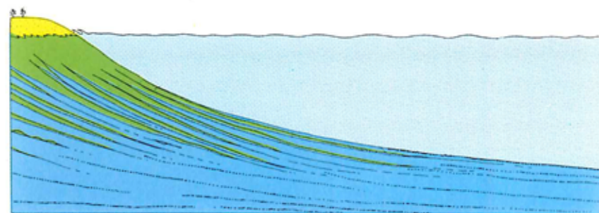
Figur 30. Aflejringsmodel for Bavnodde Grønsandet. I de dybere områder, hvor sedimentationen er ringe, ses lag af hældede knolde. Disse lag er omgivet af leret, glaukonitholdigt finsand, der ofte er helt gennemgravet. De sandede stormsandslag strækker sig ud i de dybere områder, men der er flere af dem tæt ved kysten. Efter W. Bruch, 1984.
