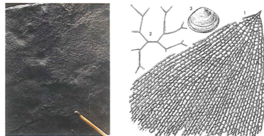
Figur 21. Lagflade i skifer med netværk af Rhabdinopora (tidligere henregnet til Dictyonema ). Til højre ses 1. ' Dictyonema ' og fra den øvre del af skiferen 2. graptoliten Clonograptus og 3. brachiopoden Broeggeria . Foto: Ole Bang Berthelsen. Tegning: Christian Rasmussen.
