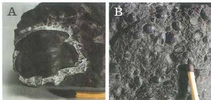
Figur 12. Trilobiter fra Mellem Kambrium. A. Paradoxides (hoved) fra 'Exsulans Kalken'. En anden art af Paradoxides fra den øvre del af Nedre Alunskifer kan blive 3 gange større, men findes kun som fragmenter. B. Ptychagnostus (hoveder og haler) fra toppen af Nedre Alunskifer. Foto: Ole Bang Berthelsen.
