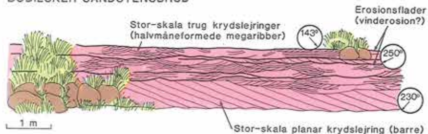
Figur 3. Profilskitse fra det sydøstlige hjørne af Bodilsker Sandstensbrud. De indcirklede tal angiver gennemsnit af strømretningsmålinger for bænkerne.
