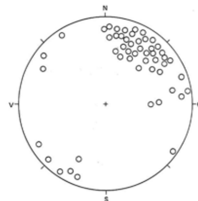
Figur 3. Den målte orientering af af-lange sten i moræneleret. Målingerne viser en koncentration i den nordøstlige kvadrant og angiver således, den retning isen kom fra. Punkter tæt ved periferien angiver sten med ringe dyk, mens punkter nær centrum angiver sten, der har et stort dyk.
