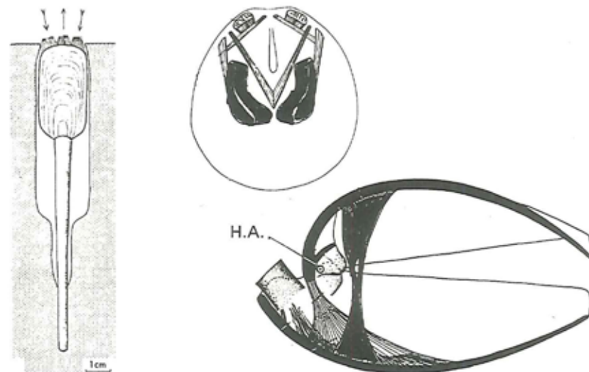
Figur 1. Til venstre ses Lingula i livsstilling. Øverst til højre ses musklerne hos den hængseløse Crania. Dorsalskallen er fjernet. Nederst til højre er der et længdesnit af Terebratulida. H.A. er hængselaksen, sort er lukkemuskler og stribet er åbnemuskl., skræmmuskler og stilkfæstningsmuskler. Hos de hængseløse brachiopoder bruges skræmmusklerne til at rotere skallerne i forhold til hinanden, så uønsket sediment slynges bort. Hos de hængslede former har stilmusklerne samme funktion, idet dyret kan rotere i små ryk om stilken.
