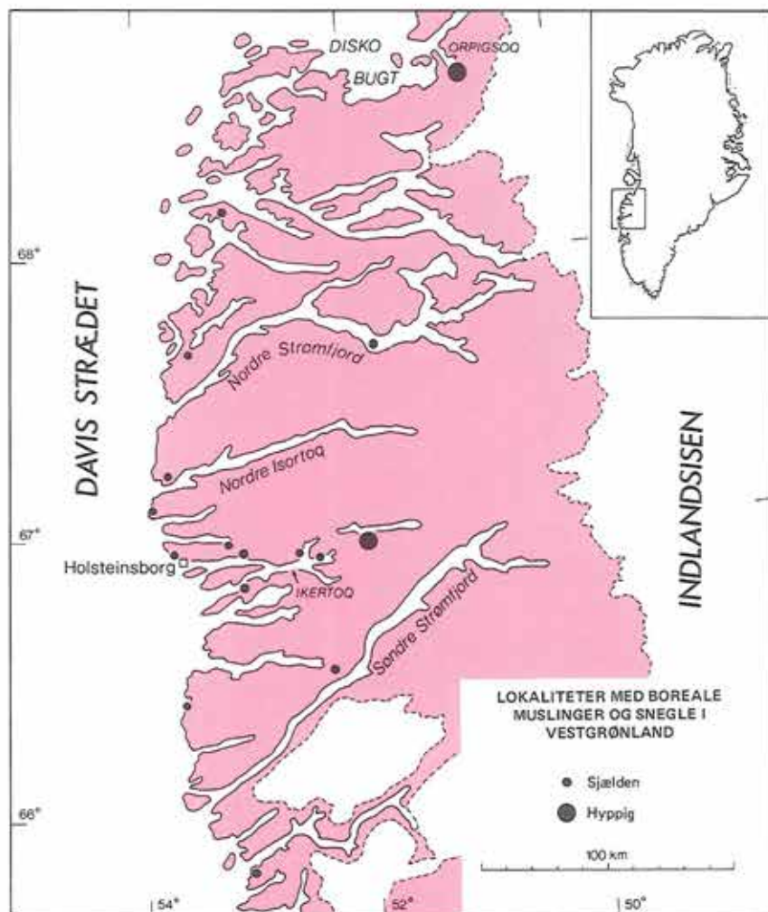
Figur 6. Udbredelsen af boreale, nu uddøde muslinger og snegle i Grønland. De boreale arter findes kun i et område mellem 65°30' og 68°30' N og kun ved yderkysterne og i korte fjorde.
