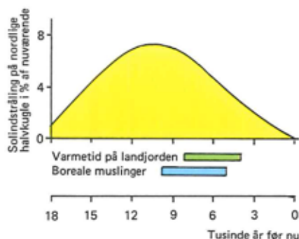
Figur 1. Kurve over orbitale ændringer i solindstrålingen på den nordlige halvkugle i de sidste 18.000 år angivet i procent af den nuværende indstråling. Kurven viser, at sommerindstrålingen toppede for lidt mere end 9000 år siden. De boreale muslinger indvandrede til Vestgrønland umiddelbart efter maksimum for solindstrålingen, mens opvarmningen på landjorden først indtraf ca. 1000 år senere.
