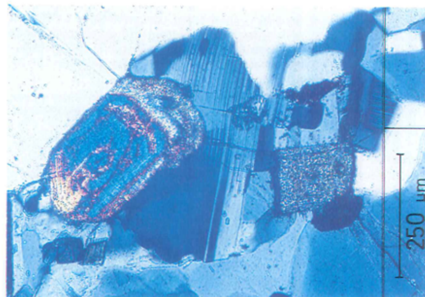
Figur 8. Nærbillede af zirkonen, der er vist i figur 7. Zirkonkrystallen viset tydelig zonar opbygning. Det omliggende mineral er feldspat, der kendes på tvillinglamellerne. Billedet er optaget med krydsede nicoller.
