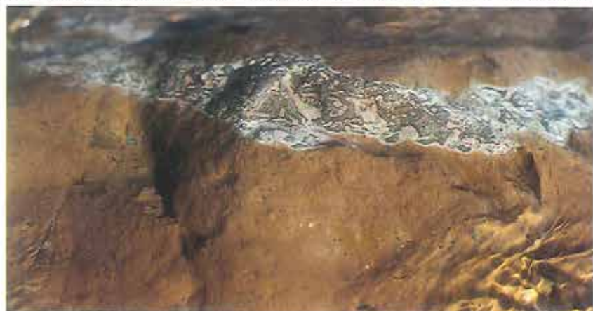
Figur 14. Røsnæs Lerets bundlag i strandkanten ud for 11 meter mærket. Det mørke lag med hvide gravegange er et 2 cm tykt askelag. Spredt i det rødbrune ler ses mindre mørke pletter. Nogle af disse er glaukonitkorn, andre er muligvis omlejrrede småklumper fra Ølst Formationen.
