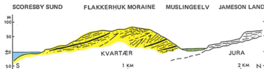
Figur 3. Skematisk snit gennem Flakkerhuk morænen. De tykke sorte lag er morænelag (till). I øvrigt opbygges ryggen af tidevandsprægede marine sedimenter.
