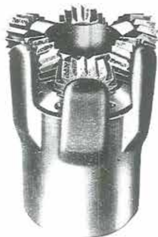
Figur 5. Borekrone med rullemesler.
