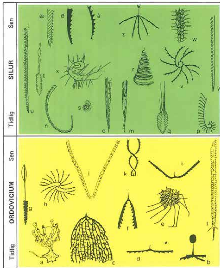
Figur 4. Diagram som viser graptoliternes mangeartede koloniformer gennem Ordovicium og Silur. a: Dictyonema (fastsiddende form). b-å: fritlevende former. b: 'Staurigrapthus', c: Rhabdinopora, d: Didymograptus, e: Loganograptus, f: Didymograptus, g: Pseudoclimacograptus, h: Nemagraptus, i: Leptograptus, j-k: Dicellograptus, l: Orthograptus, m: Akidograptus, n: Coronograptus, o: Rhaphidograptus, q og t: Petalograptus, r, s, u, x, ø og å: Monograptus, z: Linograptus. (Efter Bates & Kirk, Bulman og Müller).
