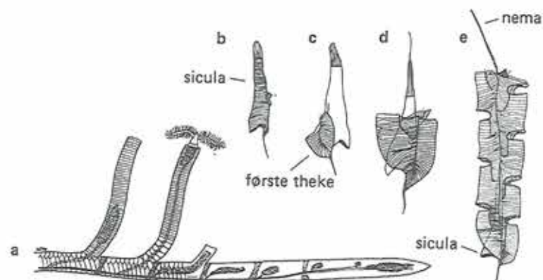
Figur 2. a: Nulevende hemichordatkoloni (Rhabdopleura), den enkelte gren er ca. 1 mm bred (efter Wienberg Rasmussen). b–e: Vækststadier af Glyptograptus, en toradet graptolit. b: Sicula, c: Sicula med den første theke, d: Det tredje theke er ved at vokse ud, e: Udvokset eksemplar (efter Mitchell).
