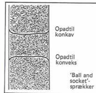
Figur 10. Skitse af tværgående 'ball and socket'-sprækkeflader.
