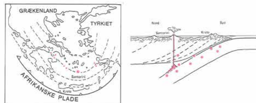
Figur 1. Kort over subduktionszonen syd for Kreta. Santorini og de øvrige vulkanske centre er vist med røde pletter. Forløbet af de Helleniske napper er vist med stiplede linier. Til højre et nord-syd gående snit gennem subduktionszonen. Her er epicentre for hyppige jordskælv vist med røde pletter.
