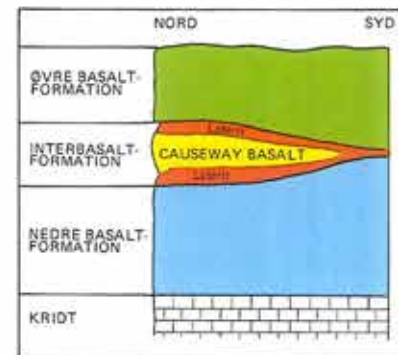
Figur 4. Placeringen af Interbasaltformationen i Antrim i forhold til Nedre og Øvre Basaltformation. 'Giant's Causeway'-lavstrømmene er begrænset til den nordlige del af Interbasaltformationen, som afgrænses både øfter og nedad af tykke sekvenser af rød laterit, der er dannet ved tropisk forvitring af basalt.
