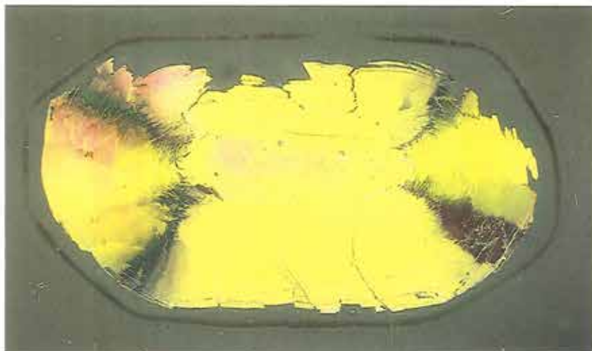
Figur 9. Tyndslib af superellipsoide (samme som i figur 8) set i polarisationsmikroskop med krydsede nicoller. Her ses subkornene som områder med lidt forskellig indbyrdes farver. De vifteformede udslukkede områder viser bøjningen i krystalgitteret.
