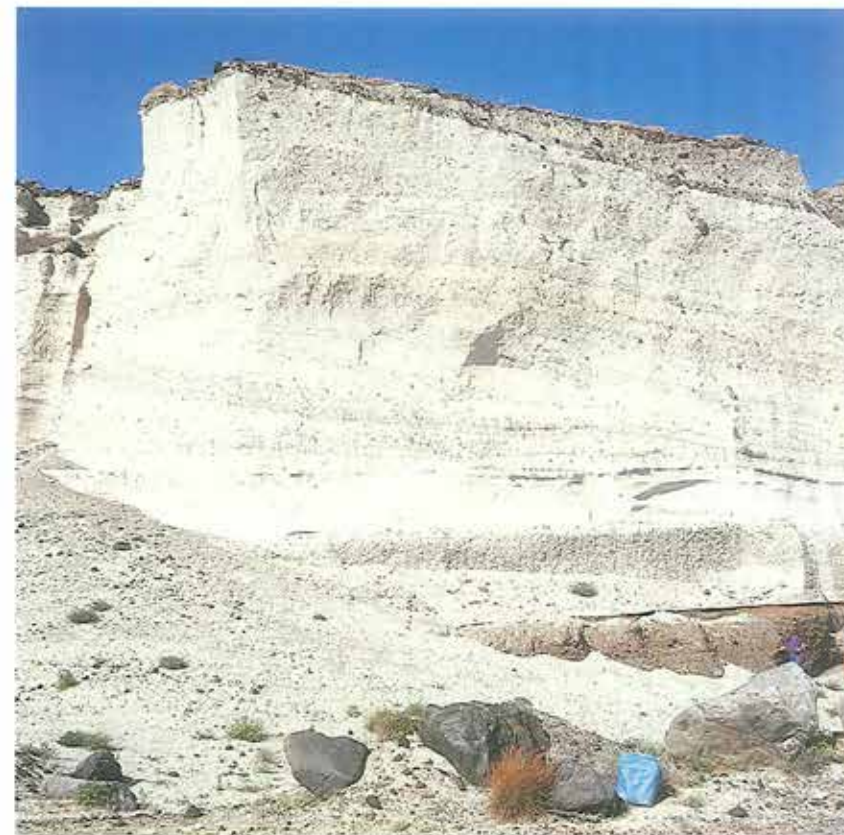
Figur 4. Askeseriens centrale del består nederst af lavvinklet, krydslejret pimpstensaske aflejret i en 'base surge' (enhed B). Herover ses den mere homogene vulkanske breccie i enhed C.
