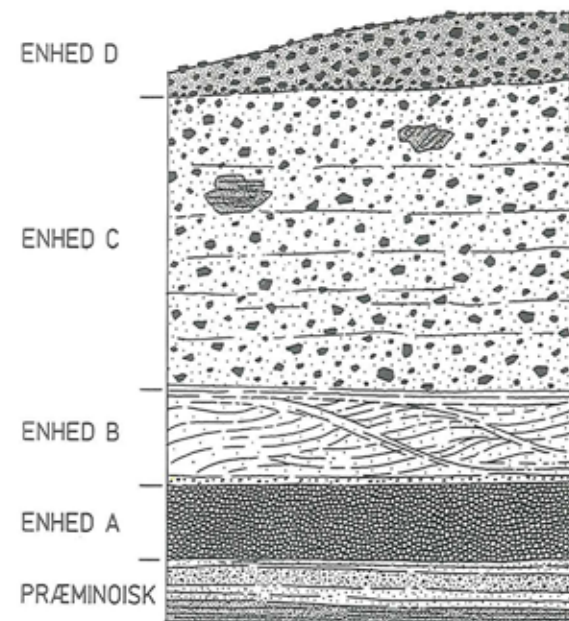
Figur 2. Profil af det Minoiske pimpstenslag på Santorini. Aflejringen kan tydeligt inddelges i 4 enheder, der hver svarer til en vulkanologisk hændelse.
