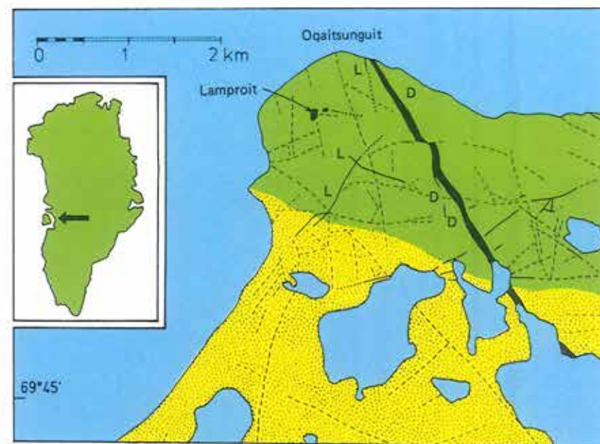
Figur 1. Kortet viser beliggenheden af lamprofyrforkomsten på forbjerget Oqaitsunguit. Grøn farve er udeformeret Atâ granit mens den gule farve er deformerede graniter og gnejer. Linier markeret med 'L' er lamprofyrgange, og linier markeret med 'D' er doleritgange.
