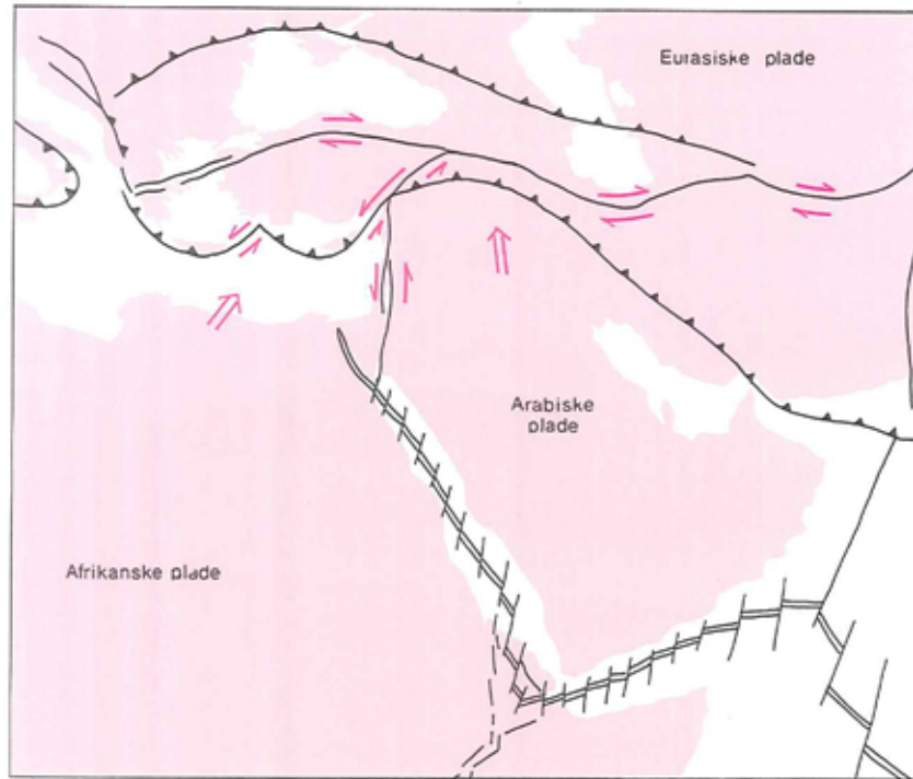
Figur 2. De overordnede relationer imellem den Afrikanske Plade, den Arabiske Plade og den Eurasiske Plade. Dobbelte pile angiver pladebevægelsen i forhold til den Eurasiske Plade, mens enkeltpile angiver den relative bevægelse langs med transforme forkastninger.
