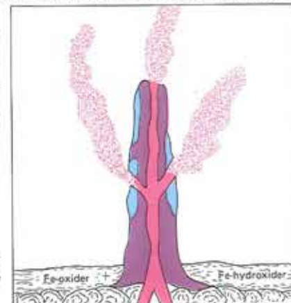
Figur 4. Opbygningen af en black smoker. Varme fluidet er rosa, sulfider er violette og sulfater blå.
