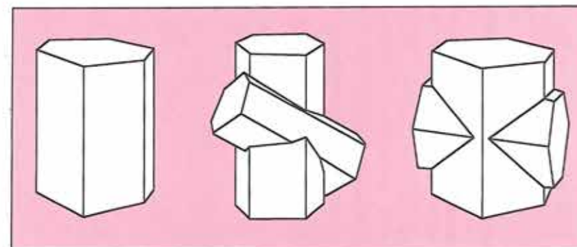
Figur 6. Skitse af perfekte staurolitkrystaller, hvoraf de to til højre er tvillingkrystaller. Mineraliet staurolit krystalliserer monoklint og danner ofte gennemvoksningstvillinger i form af et kors. Mineraliet er opkaldt efter græsk: stauros = kors og lithos = sten.
