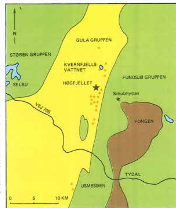
Figur 4. Forenklet geologisk kort over Selbu-Tydal-området visende nogle af møllestensbruddene (rødt). Grøn farve angiver oprindelige vulkanske bjergarter, gult omfatter oprindelige sedimentære bjergarter. Gabbro-legemet ved Fongen er vist med brun farve.
