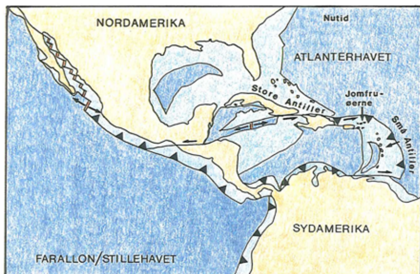
Figur 2. Rekonstruktion af pladebevægelser i det caribiske område for 100 mill. år siden. Violette områder angiver oceanbund. Bemærk, at landområders omrids er de nutidige, da det er vanskeligt at sige noget om den nøjagtige fordeling af hav og land på den tid (Kridttid).
