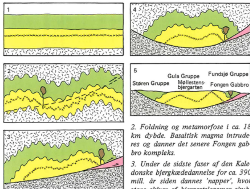
Figur 5. Den mulige geologiske udvikling i det østlige Trondheimområde.
