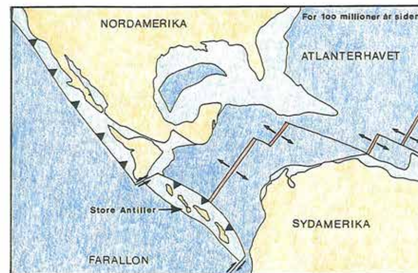
Figur 3. De nutidige aktive pladegrænser.
