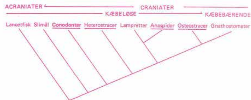
Figur 5. Stamtræ, der viser conodonerne nuværende systematiske placering blandt øvrige vertebrater. De understregede grupper er uddøde.
