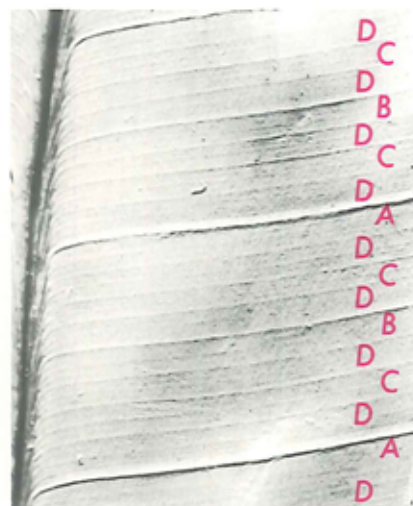
Figur 3. Nervationsmønsteret i et recent bananblad. Bemærk midterstrengen og nervations-hiraket (angivet bogstaverne A – D).
