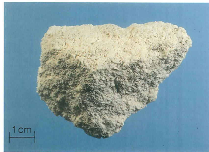
Figur 2. Bryozokalk fra Faxe Kalkbrud. Bryozokalken er opbygget af talrige små grene på under 1 mm i diameter. Bryozoerne er omgivet af finkornet kalkmudder.
