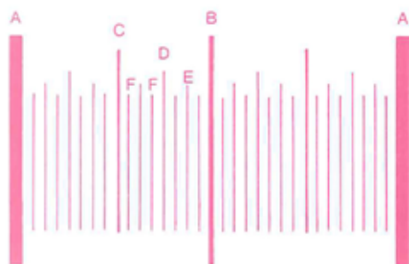
Figur 5. Skematisk billede af nervationsmønsteret udtæget fra det fossile bananblad, der ses i figur 2.
