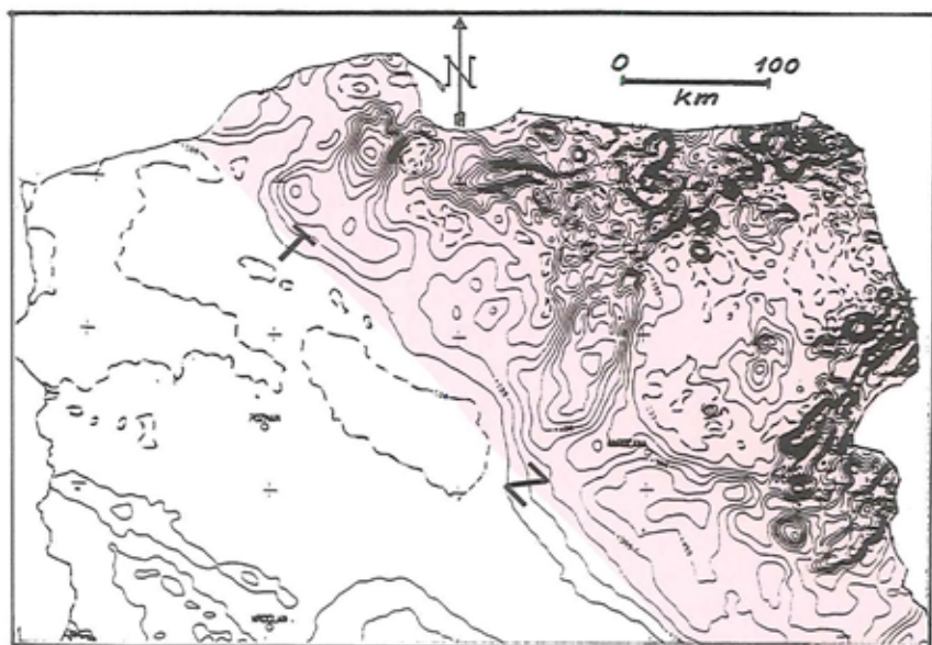
Figur 7. Moderne magnetisk kort over Polen. De fuldt optrukne, tætliggende kurver viser positive anomalier forårsaget af relativt højtliggende (mere magnetiserbart) grundfjeld under den Østeuropæiske Platform. Bemærk hvorledes de positive anomalier slutter brat langs en NV-SØ gående linie: Tornquist Linien. Efter Mapa Magnetyczna Polski (Instytut Geologiczny Warszawa).
