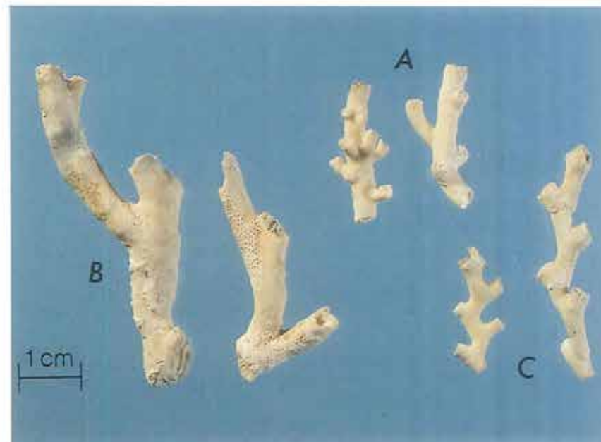
Figur 6. Fragmenter af de tre koralarter, som var de vigtigste i opbygningen af koralbankerne i Faxø Kalkbrud. A: Dendrophyllia candelabrum , der består af en hovedgren med mindre sidegrene. Opbygningen kan minde om en gammel-dags flerarmet lysestage, hvilket har givet inspiration til artsnavnet. B: Faxephyllia faxoensis er den kraftigste af de tre arter. Nye grene dannes ved at en gren deler sig i to nye, ligestillede grene. C: Oculina becki . Størrelsen varierer meget, men igen er forgreningsmønsteret karakteristisk. Kolonien er udelukkende opbygget af ensartede sidegrene, der næsten altid skifter retning. Foto: Jan Aagaard.
