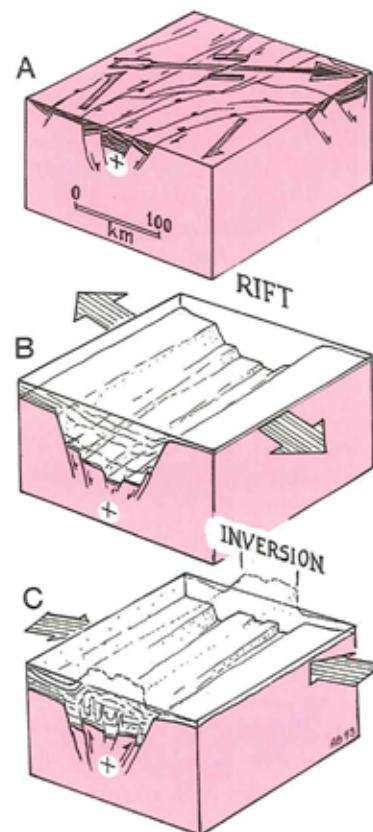
Figur 5. Forenklede blokdigrammer, der viser Tornquist Zonens udvikling.
