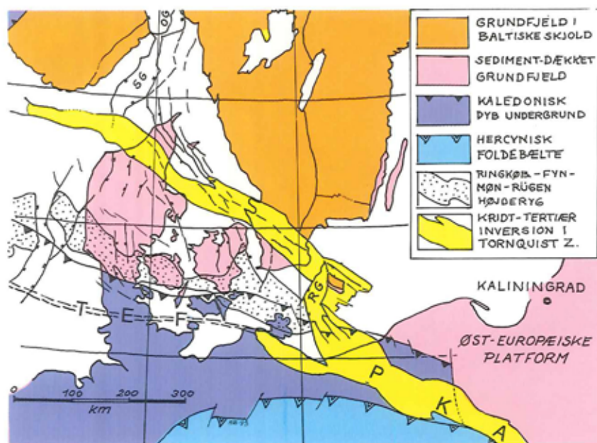
Figur 4. Undergrundens strukturer omkring Tornquist Zonen. T-E-F er den Trans-Europæiske Forkastning. SG og OG angiver Skagerrak- og Oslo gravsænkninger. I Polen kaldes den 'inverterede' (opbulede) Tornquist Zone for det Pomeranske-Kujawiske Antiklinorium (PKA).
