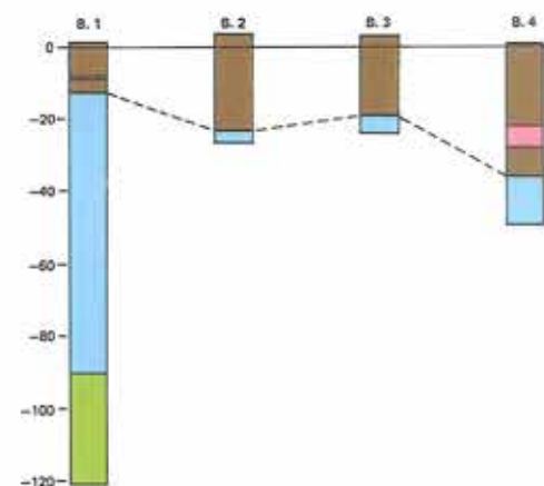
Figur 7. Hovedtræk af lagfølgerne i de fire nye undersøgelsesboringer. Lodrette skala er dybden i m. Brunt er moræner og -sand, rødt er smeltevandsaflejringer, blå farve angiver det tertiære ler med højt smectitindhold, og grønt er kalk.
