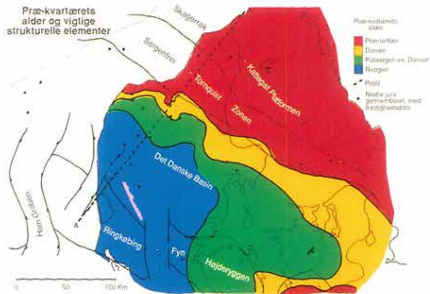
Figur 1. De præ-kvartære lags alder samt vigtige strukturelle elementer i den danske undergrund.
