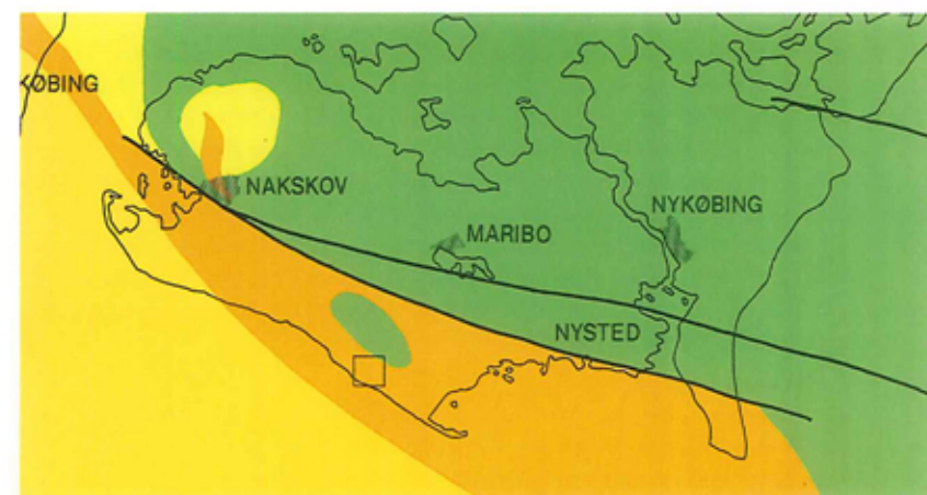
Figur 3. Formindsket udsnit af Varv's undergrundskort over Lolland og Falster. Den mørkegrønne farve angiver Øvre Kridt (skrivekridt), lysegrøn er kalk fra Danien, brunt er Paleocæne aflejringer (yngre end Danien) og lysebrunt er aflejringer fra Eocæn. Rødbyhavn-området er angivet med en firkant.
