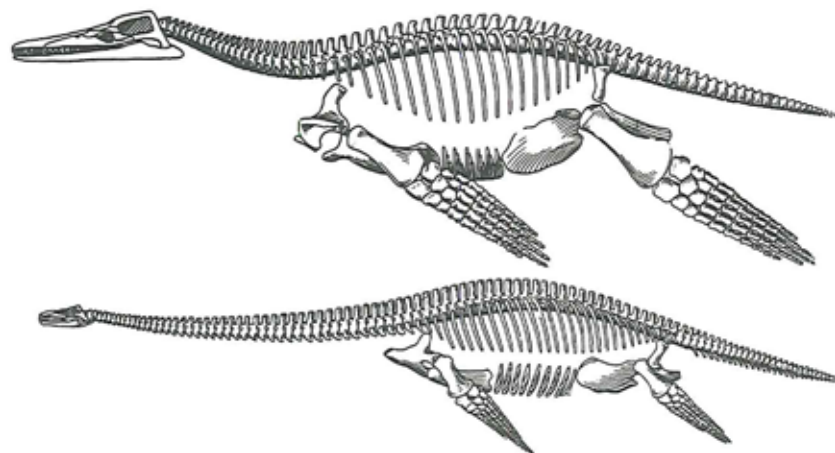
Figur 4. Rekonstruktion af to svaneøgle skeletter fra sen Jura. Øverst en kort-halset pliosaur med langt hoved og store tænder. Nederst en langhalset plesiosaur med lang hals og lille hoved. Begge skeletter er omkring 3 m lange. Rekonstrueret af Andrews, 1910.
