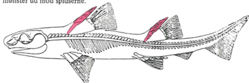
Figur 9. Rekonstruktion af Hybodus , som viser placeringen af de to pigge (røde) foran rygfinnen.
