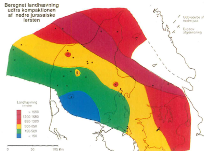
Figur 2. Beregnet landhævning på grundlag af størrelsen af kompaktionen af nede jurassiske lersten. Kompaktionen er baseret på lydmålinger i Fjerritslev Formationen.
