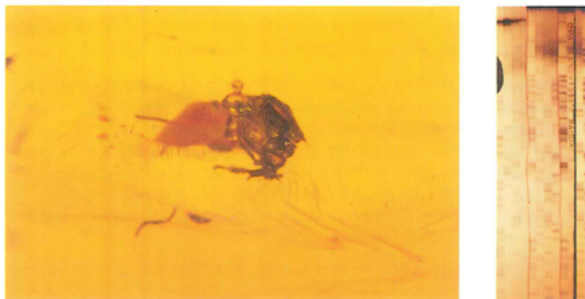
Figur 2. Dominikansk rav med en lille brodløs bi ( Probleia dominicana ), stærkt forstørret, hvorfra man har isoleret og analyseret fragmenter af DNA. Til højre ses dele af to søjler til bestemmelse af nucleotider i DNA og sammenligning mellem dem optaget på film. Foto O.B. Berthelsen
