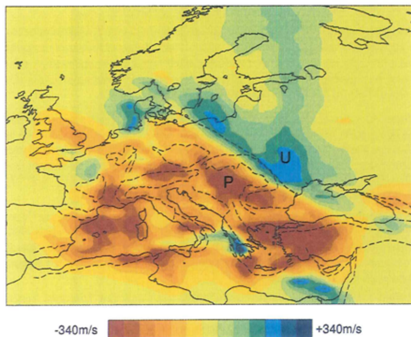
Figur 5. 'Et Tomografi af Tornquist' i 80 km's dybde, 'optaget' af A. Zielhuis, 1993. Farverne angiver områder i 80 km niveauet, hvor S-bølger med en referencehastighed af 4500 m/s (gult) får formindsket (-340 m/s: rødt) eller forøget (+340 m/s: blå) deres hastighed. De brudte sorte streger viser vigtige tektoniske grænser.
