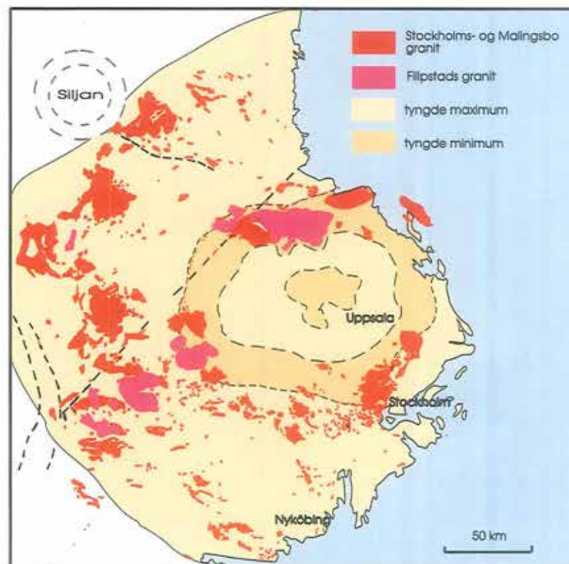
Figur 5. Upplandsstrukturen ses som en central tyngdeanomali omgivet af meget fragmentrige magmatiske bjergarter, som går under betegnelsen Stockholms- og Malingsbogrinit.
