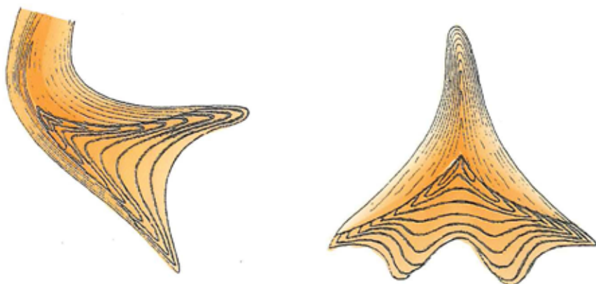
Figur 2. Tværsnit af conodoner med lamellar opbygning. Det organiske materiale der bliver farvet, findes langs lamellerne og inde i conodonerne.
