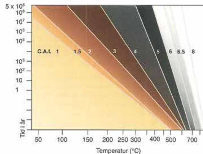
Figur 3. Arrhenius diagram. Ved hjælp af diagrammet omsættes CAI-værdier til temperaturintervaller.
