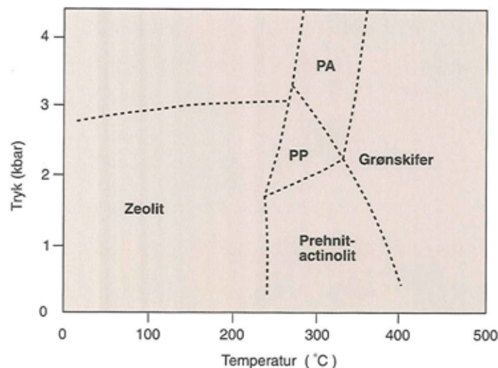
Figur 5. Lavmetamorfe facies og deres tryk- og temperaturfelter.
